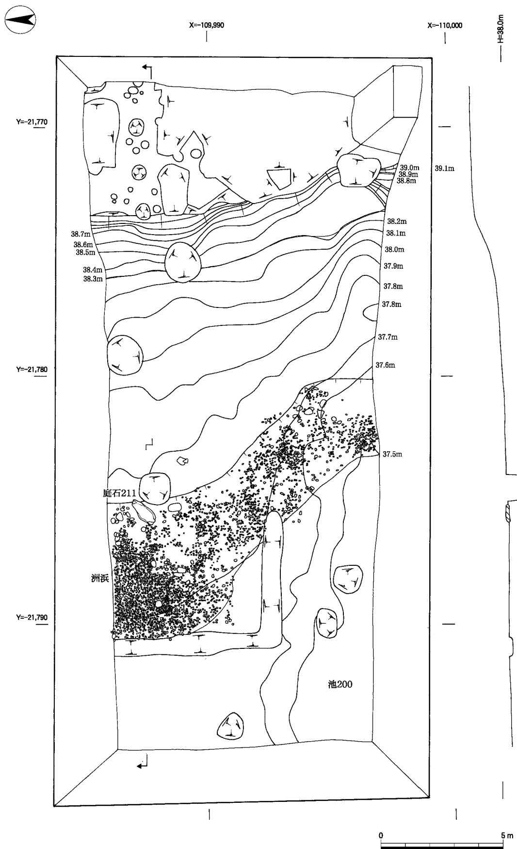
第5面遺構実測図(1:150)
