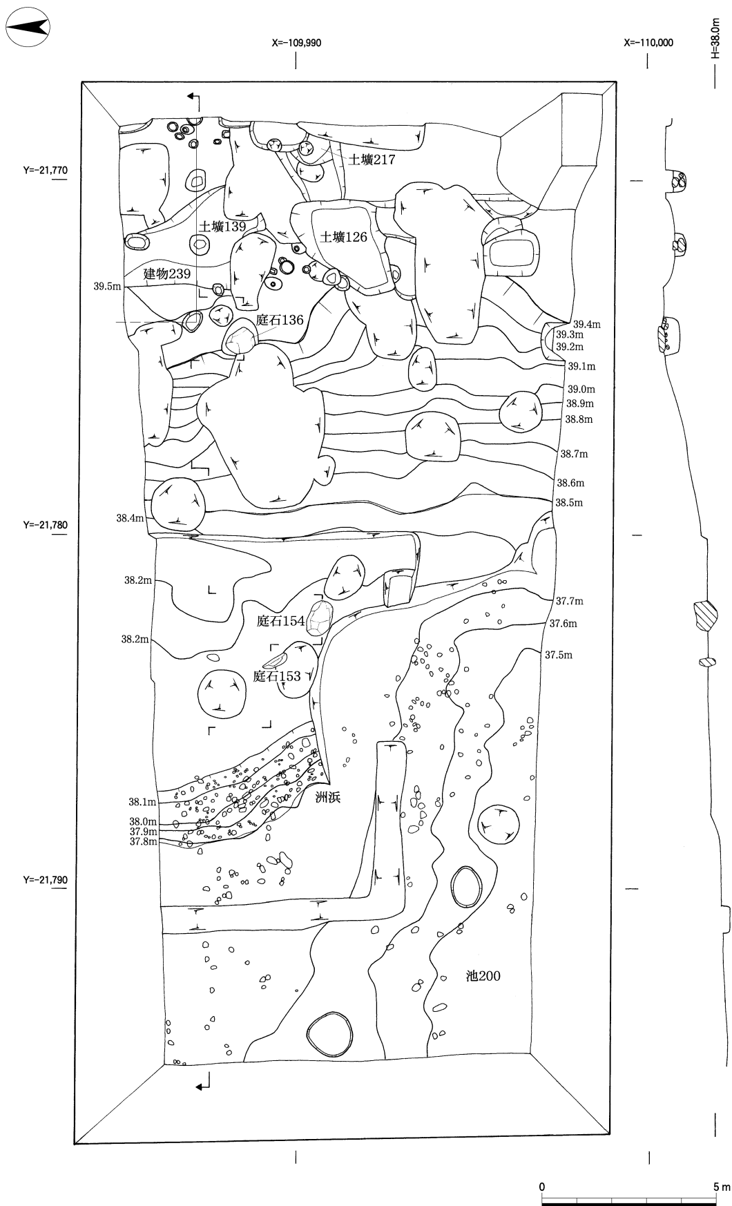
第3面遺構実測図(1:150)
