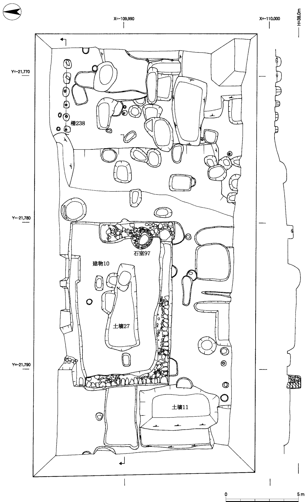
第1面遺構実測図(1:150)
