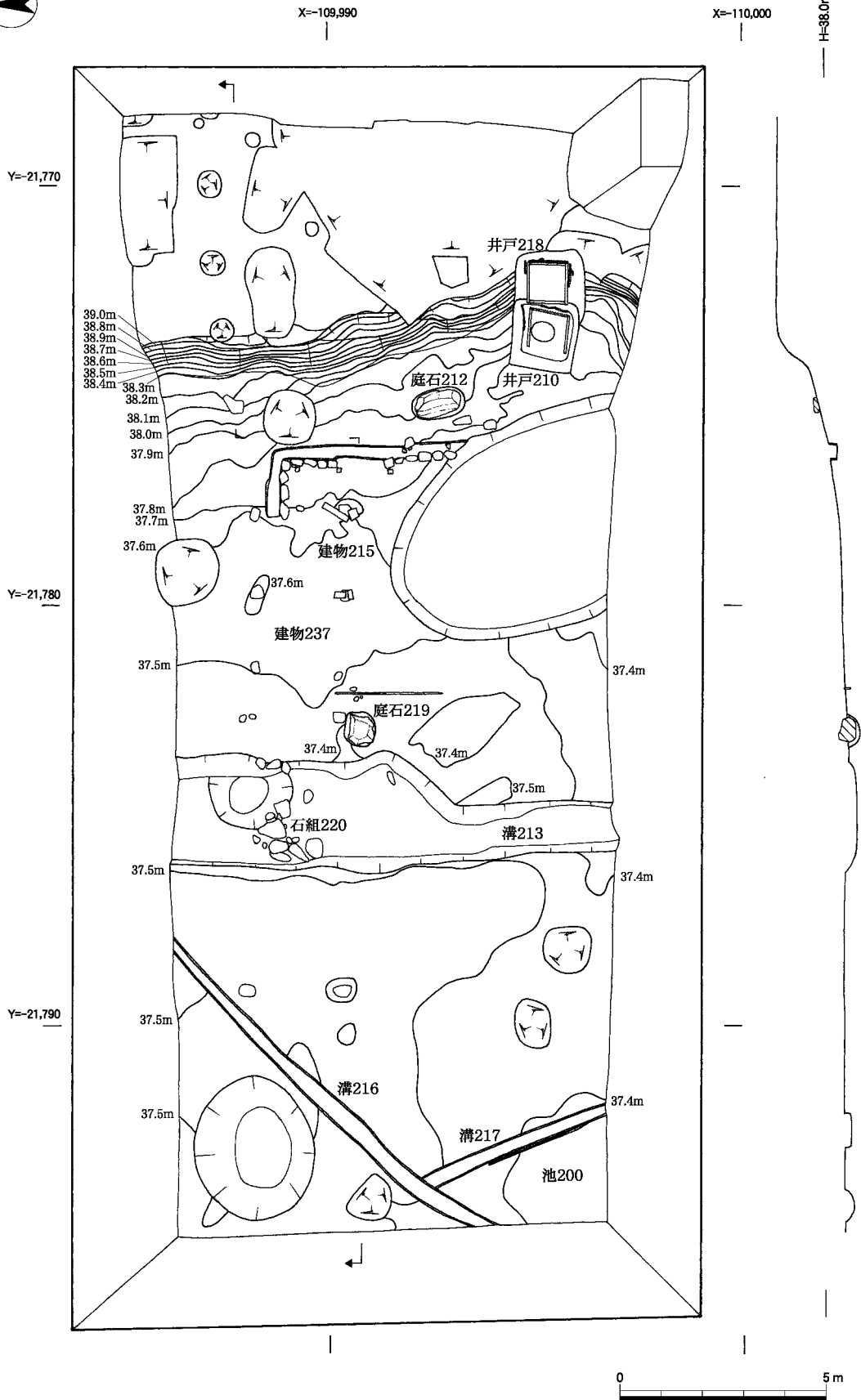
第6面遺構実測面図 ( 1 : 150 )
