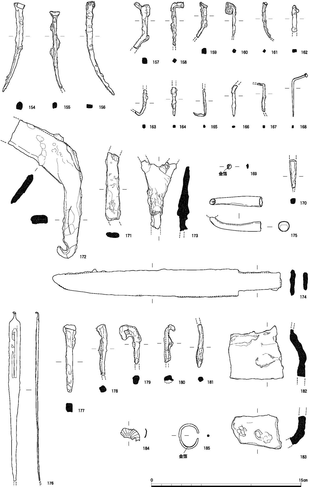
金属製品実測図 ( 1 : 2 )
