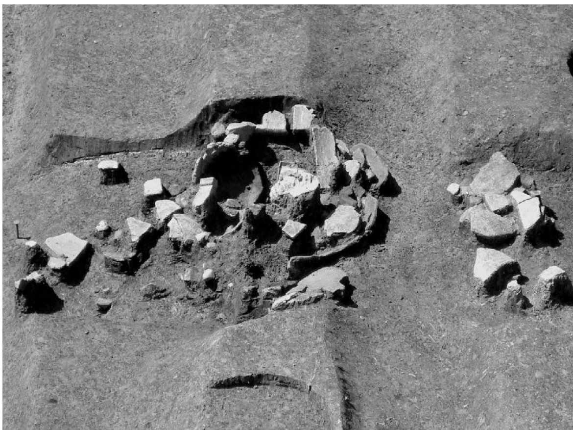
1 南調査区土坑2 (北から)
