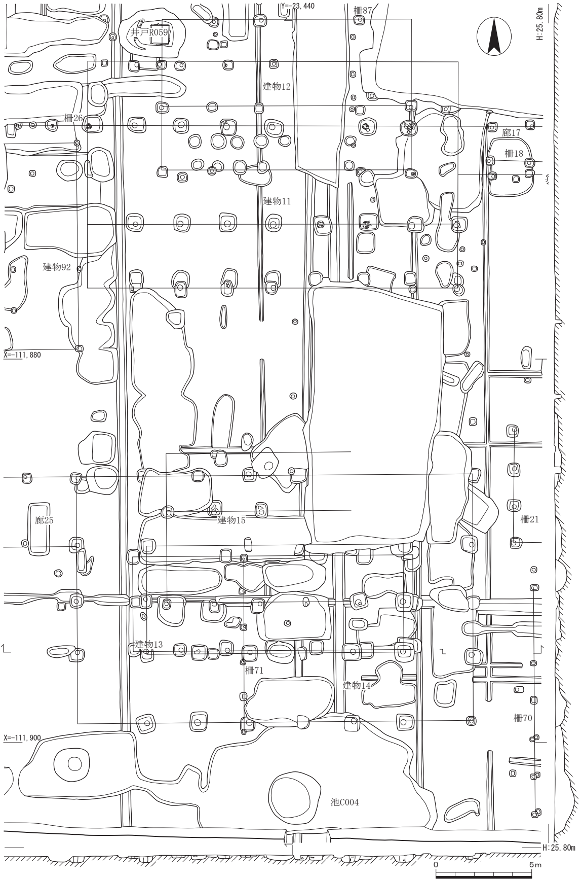
遺構図
