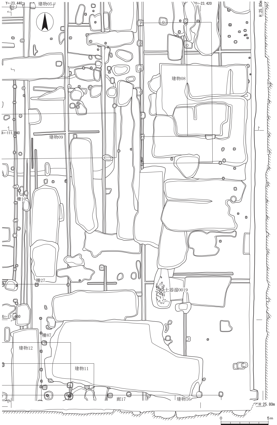
遺構図
