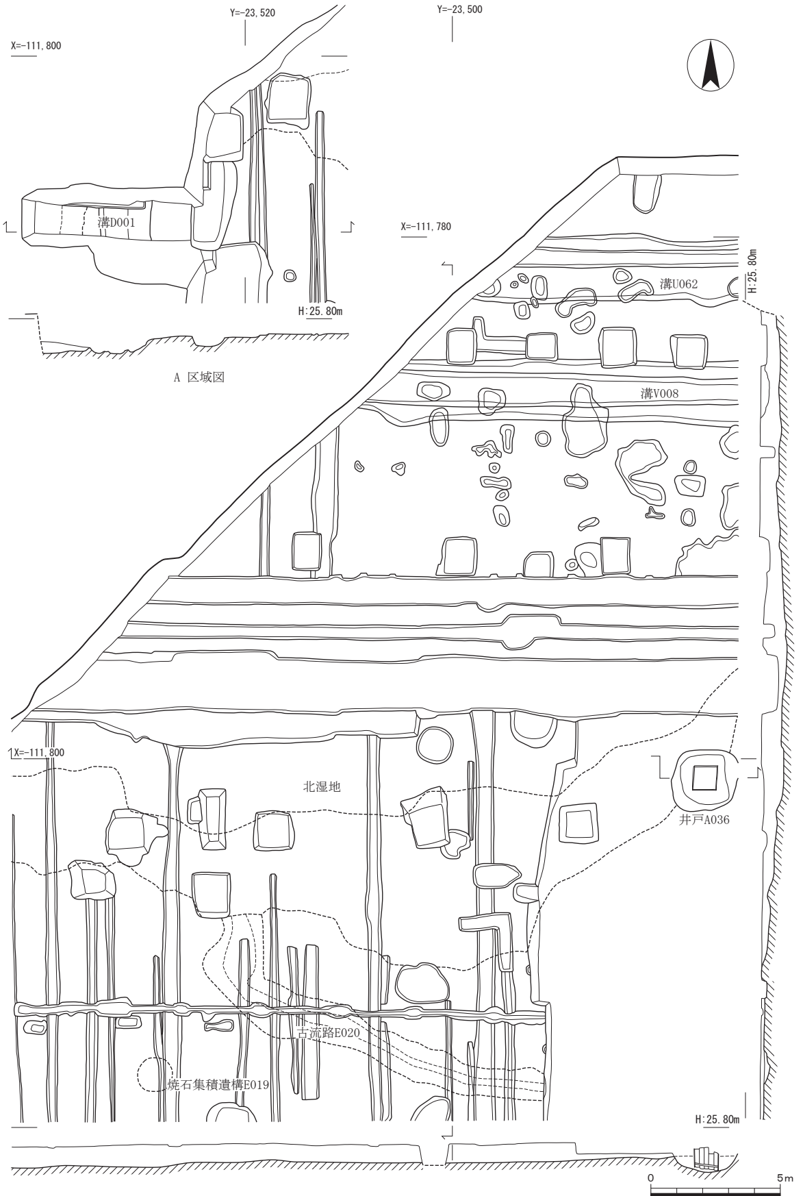
遺構図
