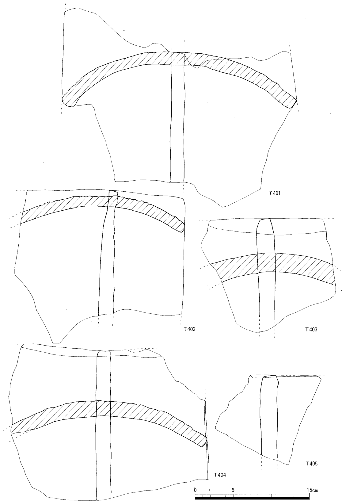
平瓦 (1:3)
