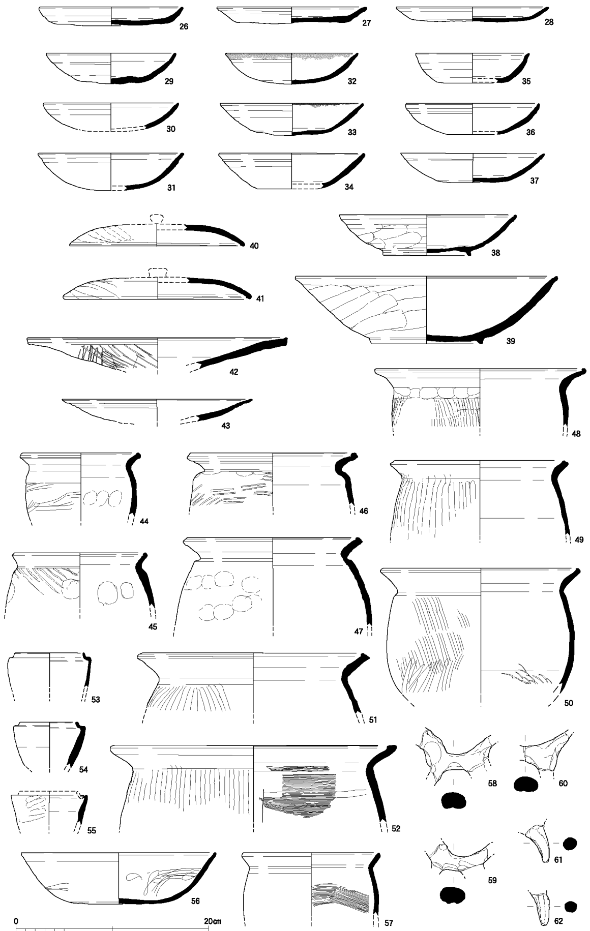
7次調査5区出土土器実測図(1:4)
