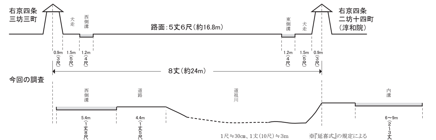
図8 道祖大路・道祖川の断面模式図(1:200)
