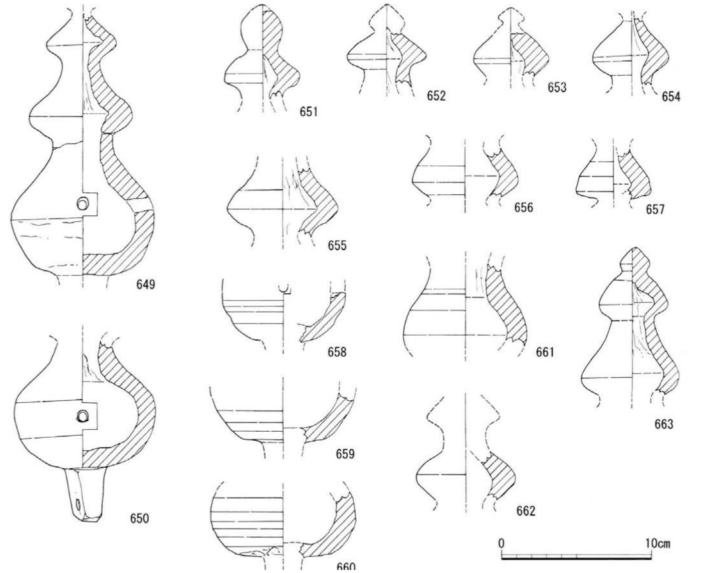
ひさご形土製品実測図
