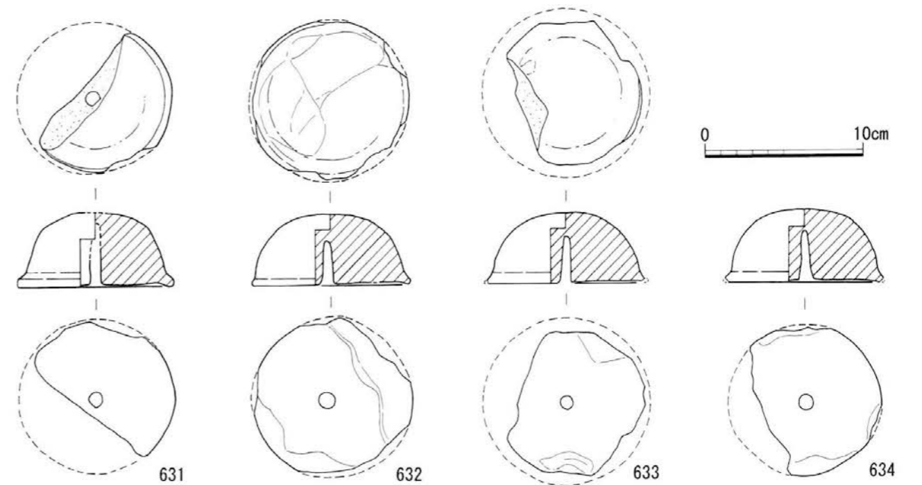
覆鉢形土製品実測図
