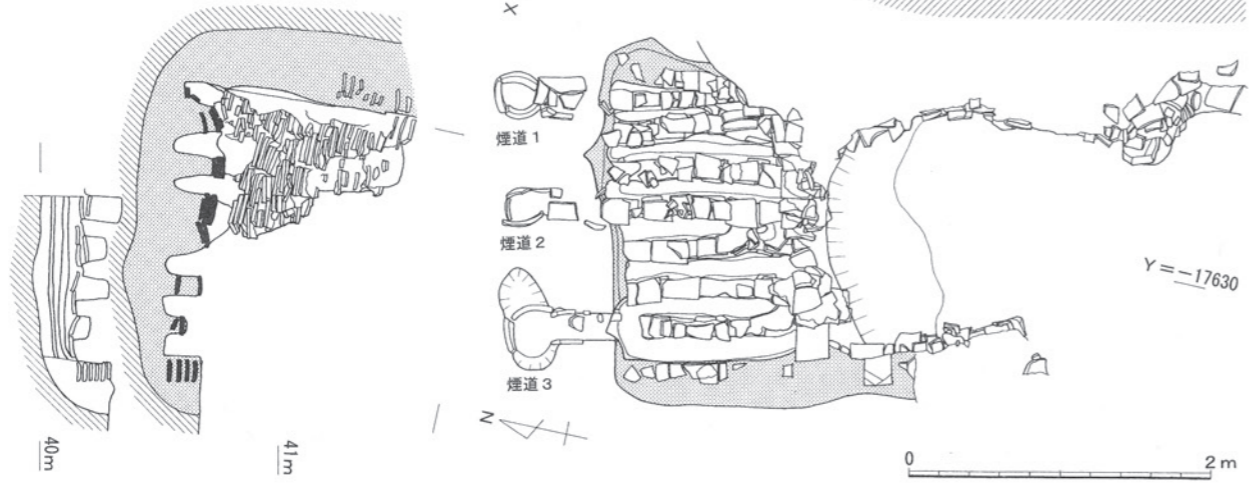
図5 法琳寺瓦窯遺構平面・断面図 (1:50)
