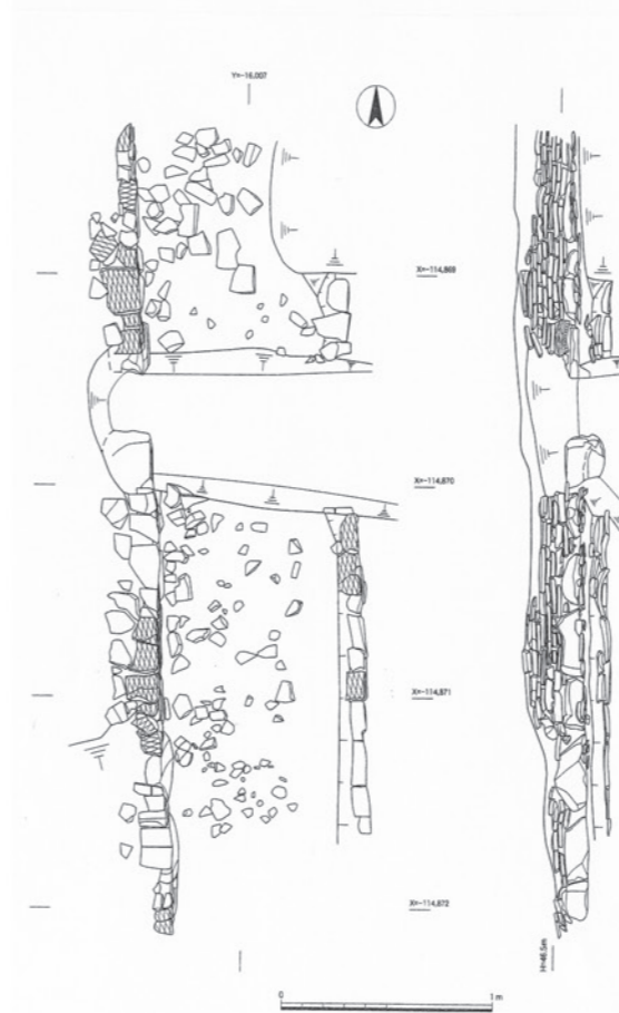
図11 平成16年度調査瓦積二重基壇平面および見通し図 (1 : 40)
