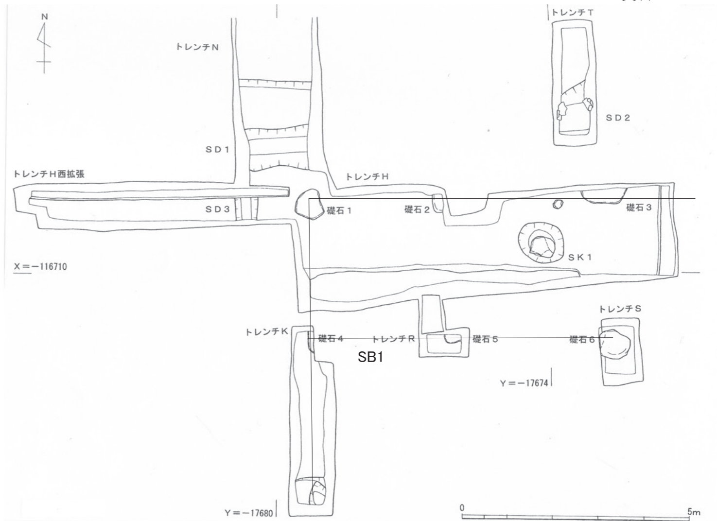
図3 建物SB1遺構平面図 (1:80)
