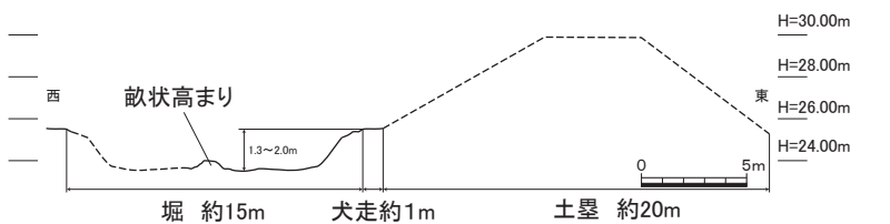
図6 JR丹波口駅周辺調査からの御土居復元模式図(1:400)
