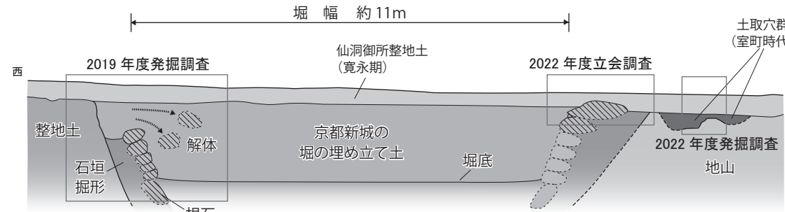
図14 京都新城堀の埋没過程模式図
