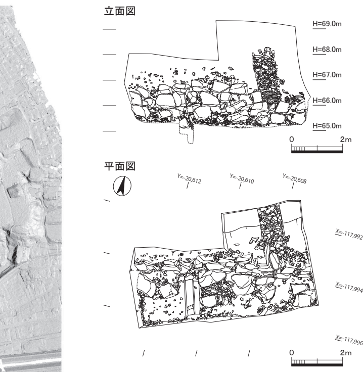
図12 2022年度検出石垣平面・立面図(京都市文化財保護課2023より転載)(1:150)
