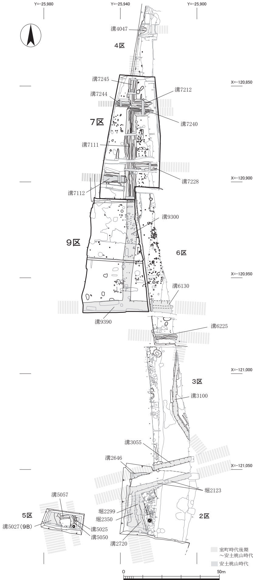
図8 淀水垂大下津遺跡堀状遺構図(室町時代後期から安土桃山時代、1:1,200)
