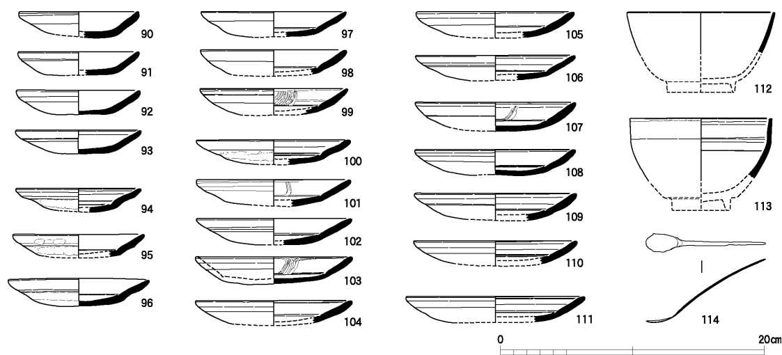
図14 東区SK44下層出土土器・金属製品実測図（1：4）
