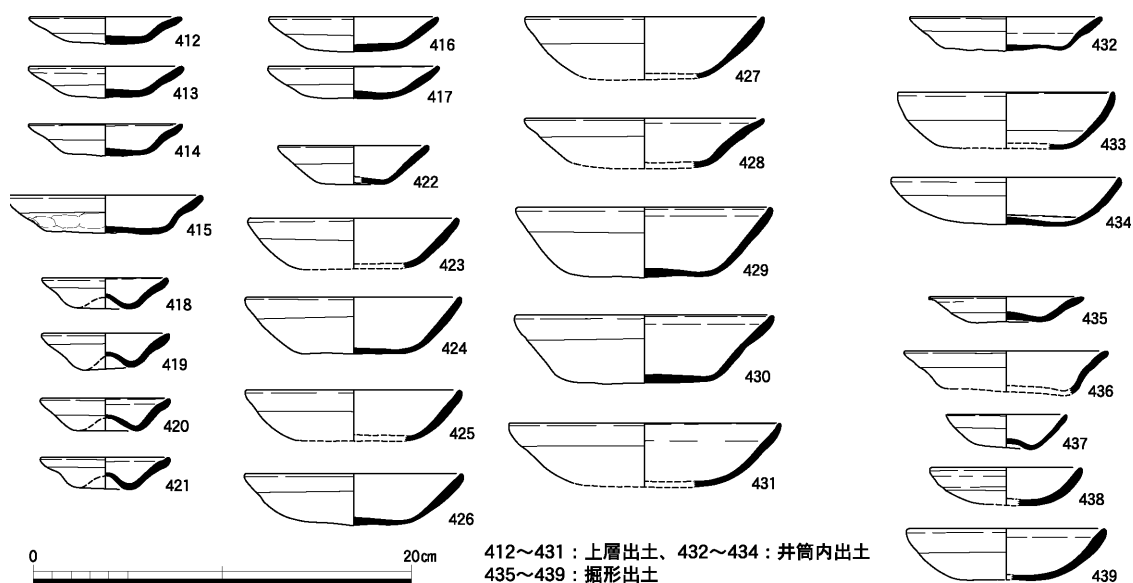
図20 東区SE211出土土器実測図（1：4）
