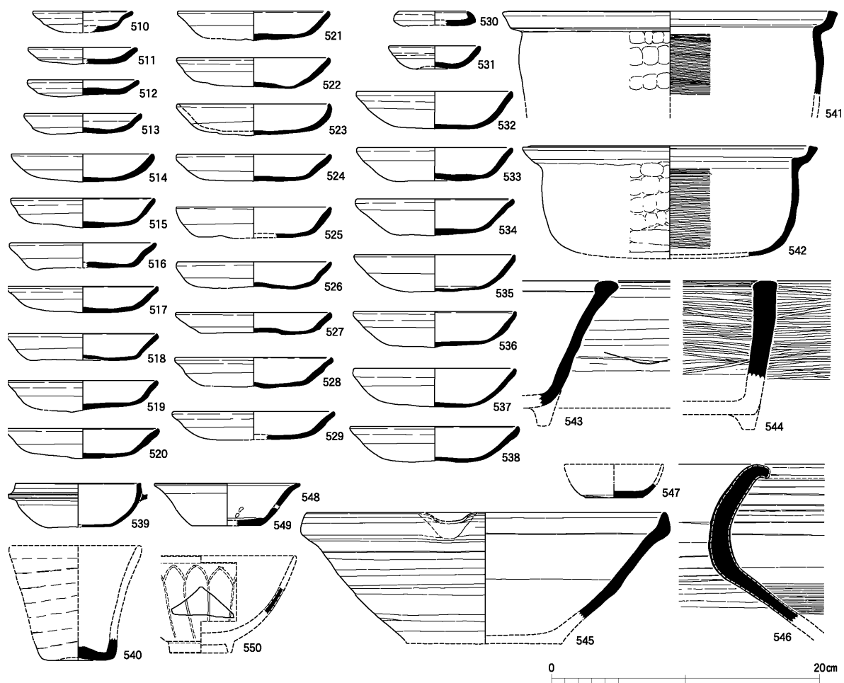
図22 西区SK51下層出土土器実測図（1：4）
