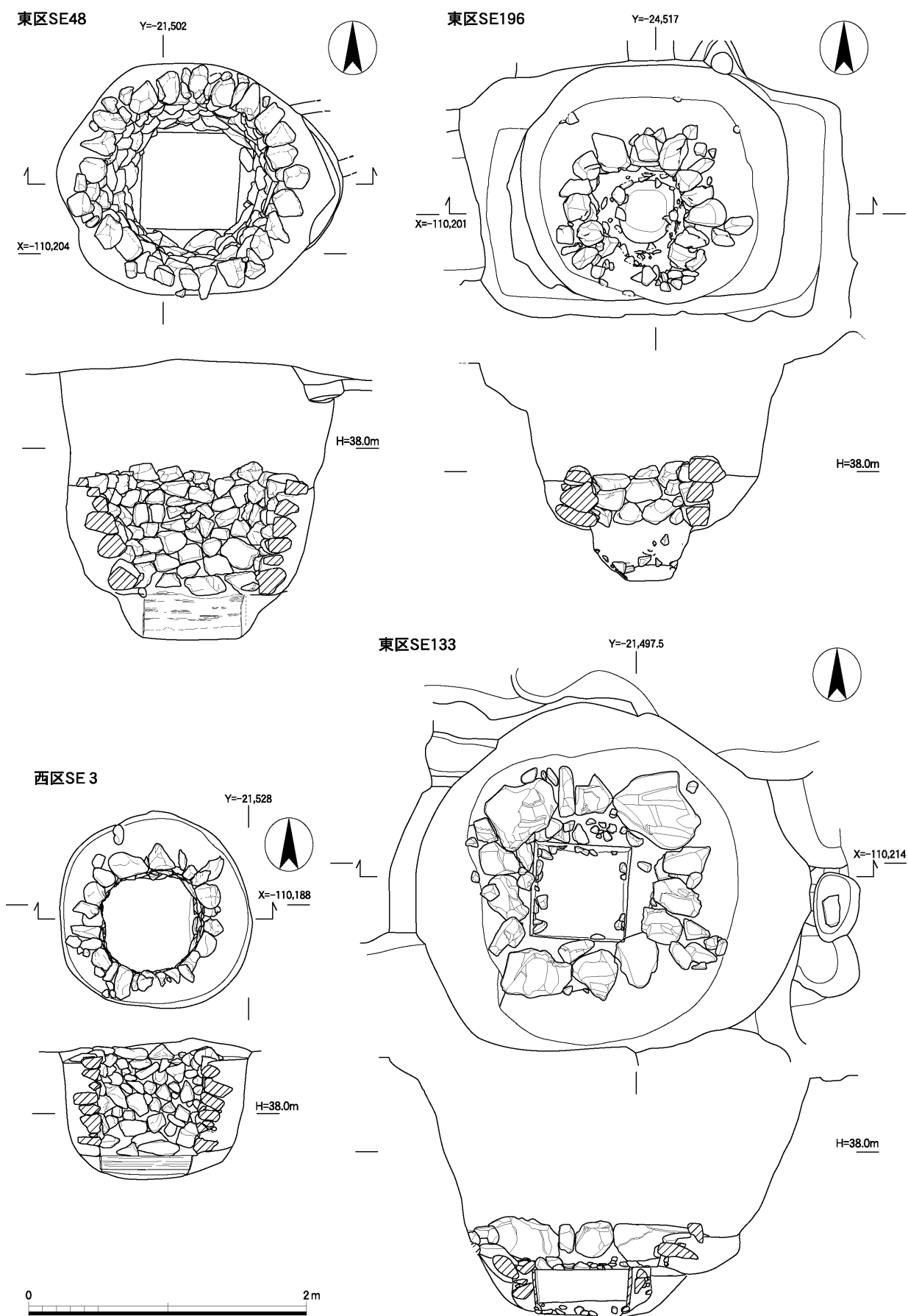
图7 東区SE48・133・196、西区SE 3实测图（1：40）
