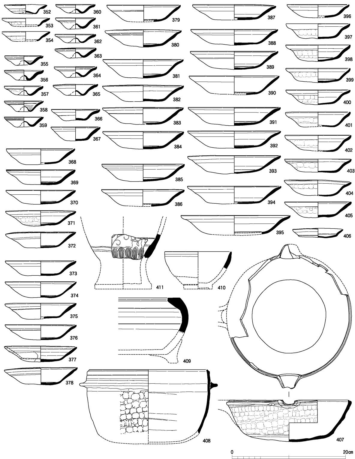
図19 東区SE238中層出土土器実測図（1：4）
