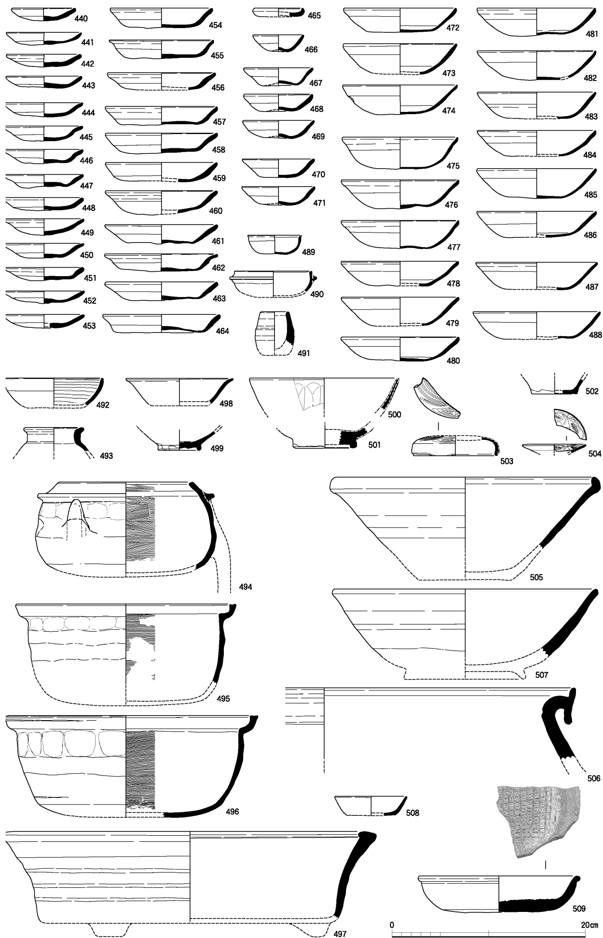
图21 西区SK51中層出土土器实测图（1：4）
