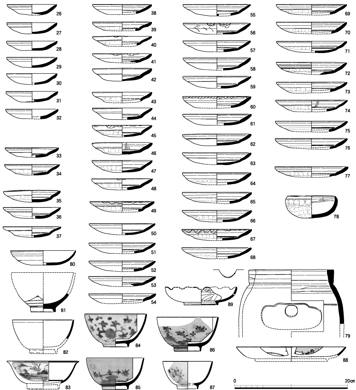
図13 東区SK44炭層出土土器実測図（1：4）
