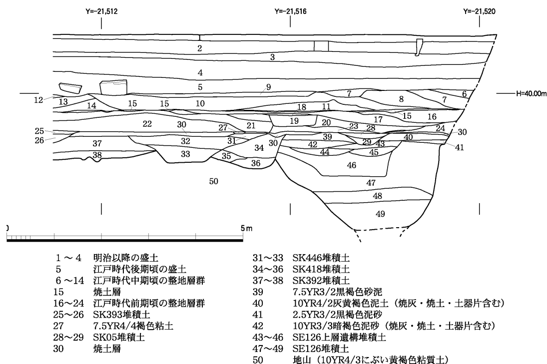
図4 東区南壁断面図（1：80）
