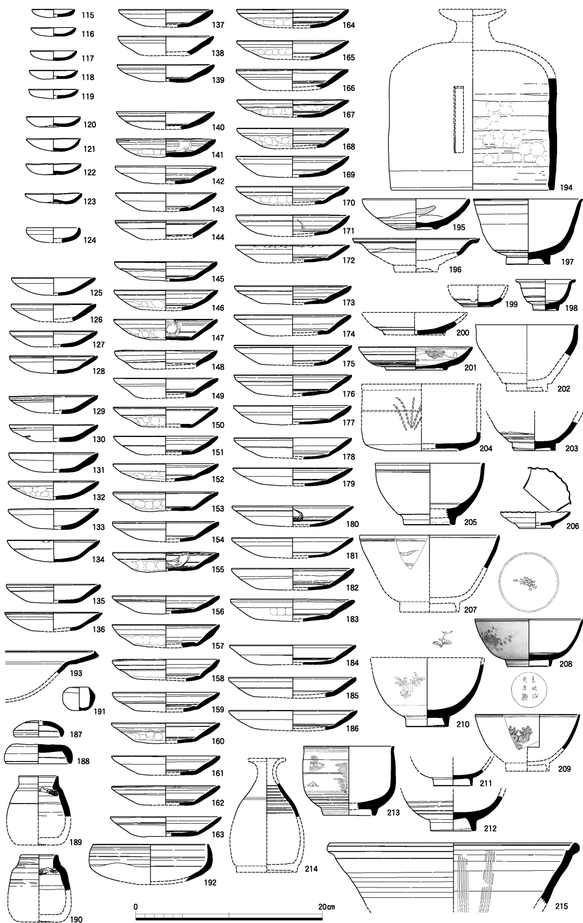
图15 东区SK51上段出土土器实测图（1：4）
