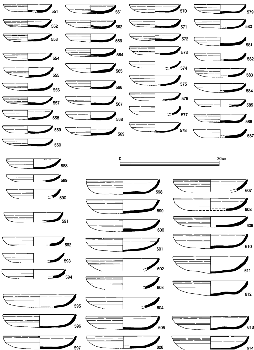
図23 東区SK419出土土器実測図（1：4）
