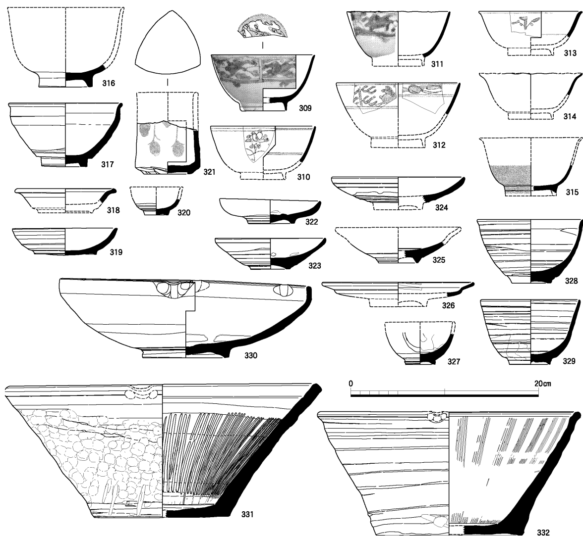
图17 东区SK51下段出土土器实测图 2 (1 : 4)
