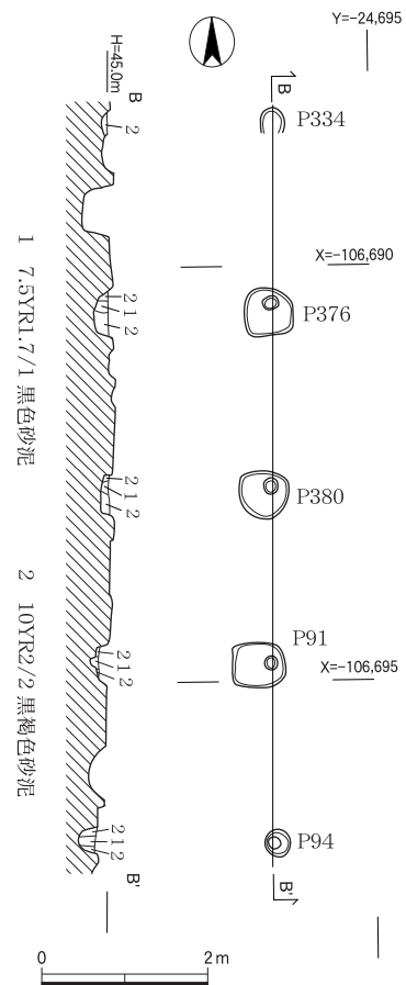
图11 柵3実測図（1：100）
