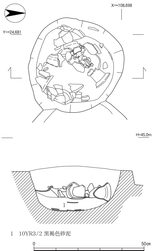
図17 土壌235実測図（1：10）
