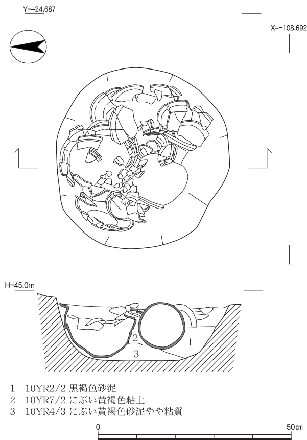
図18 土壌300実測図（1：10）
