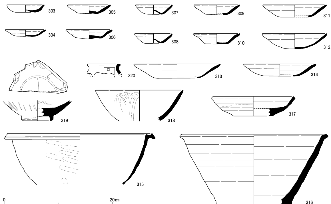
土器実測図6 (1:4)
