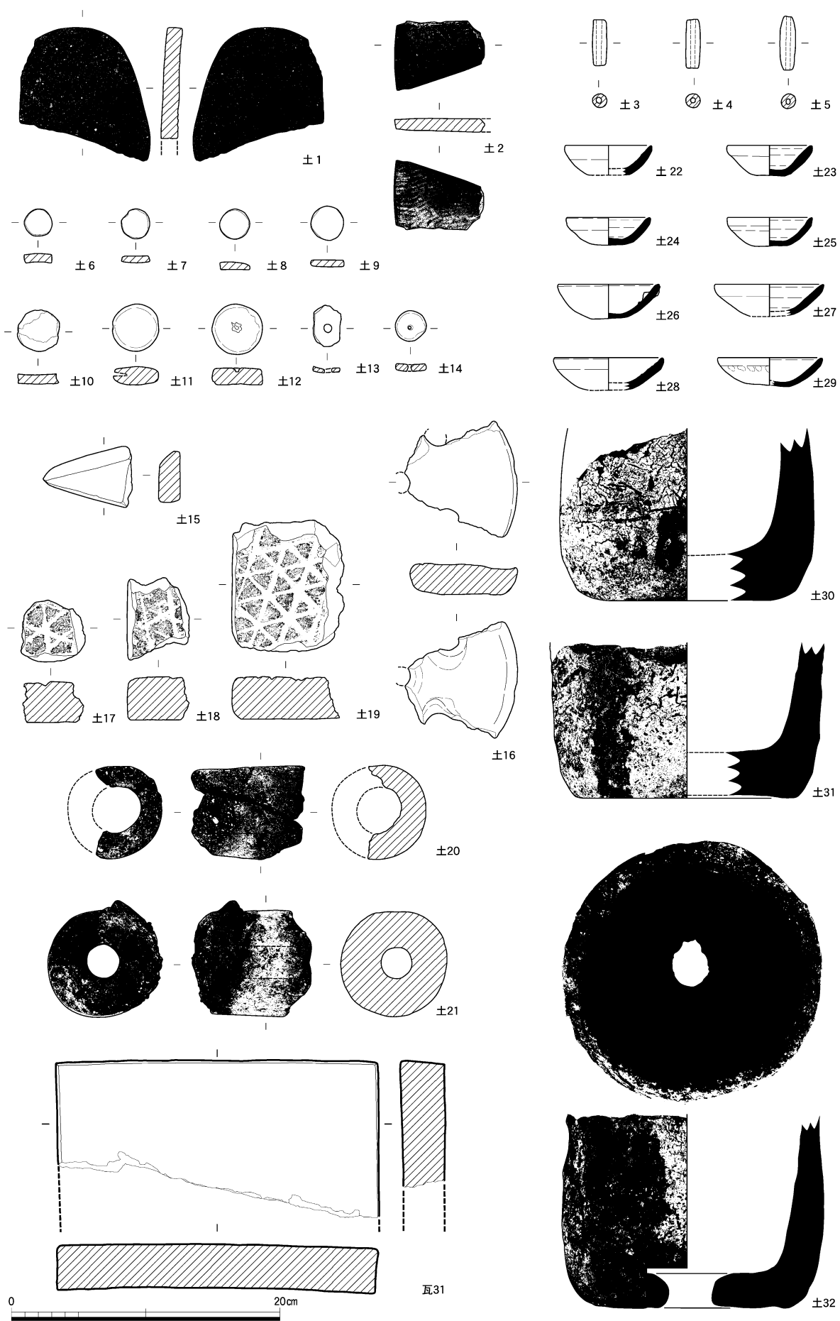
瓦類実測図3、土製品実測図1 (1 : 4)
