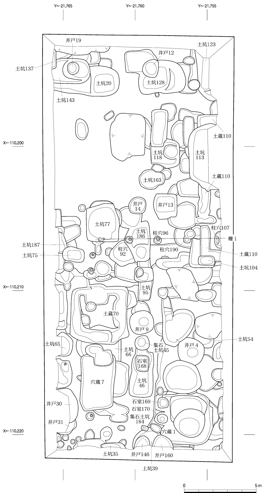
2区第1面遺構平面図 (1 : 150)
