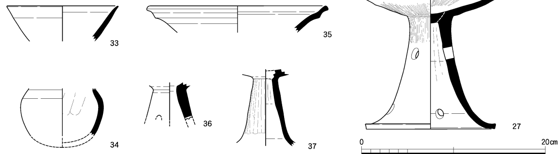
土器実測図1 (1:4)
