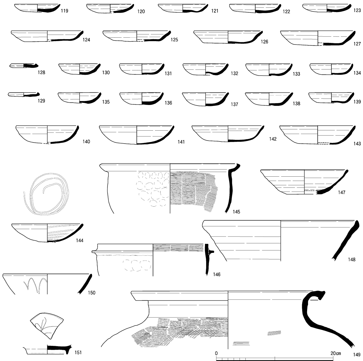
土器実測図3 (1:4)
