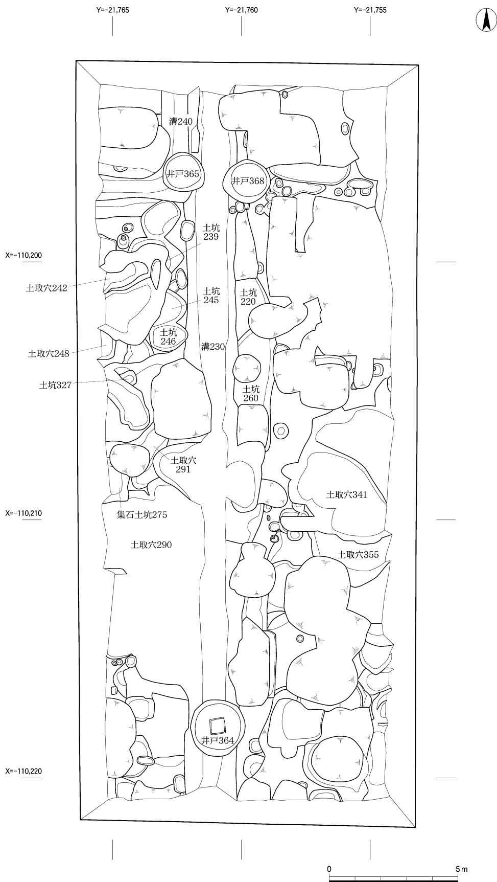
2区第2面遺構平面図 (1 : 150)
