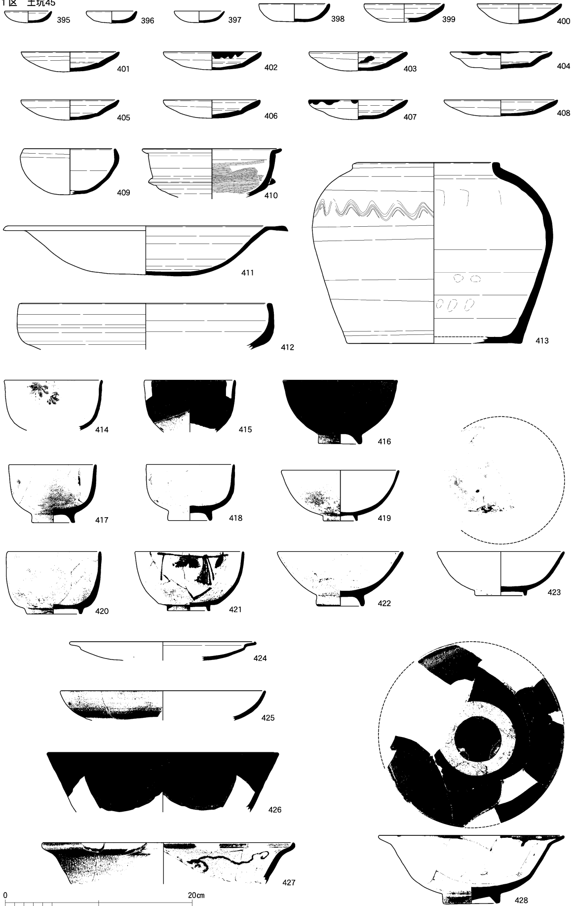
土器実測図9 (1:4)
