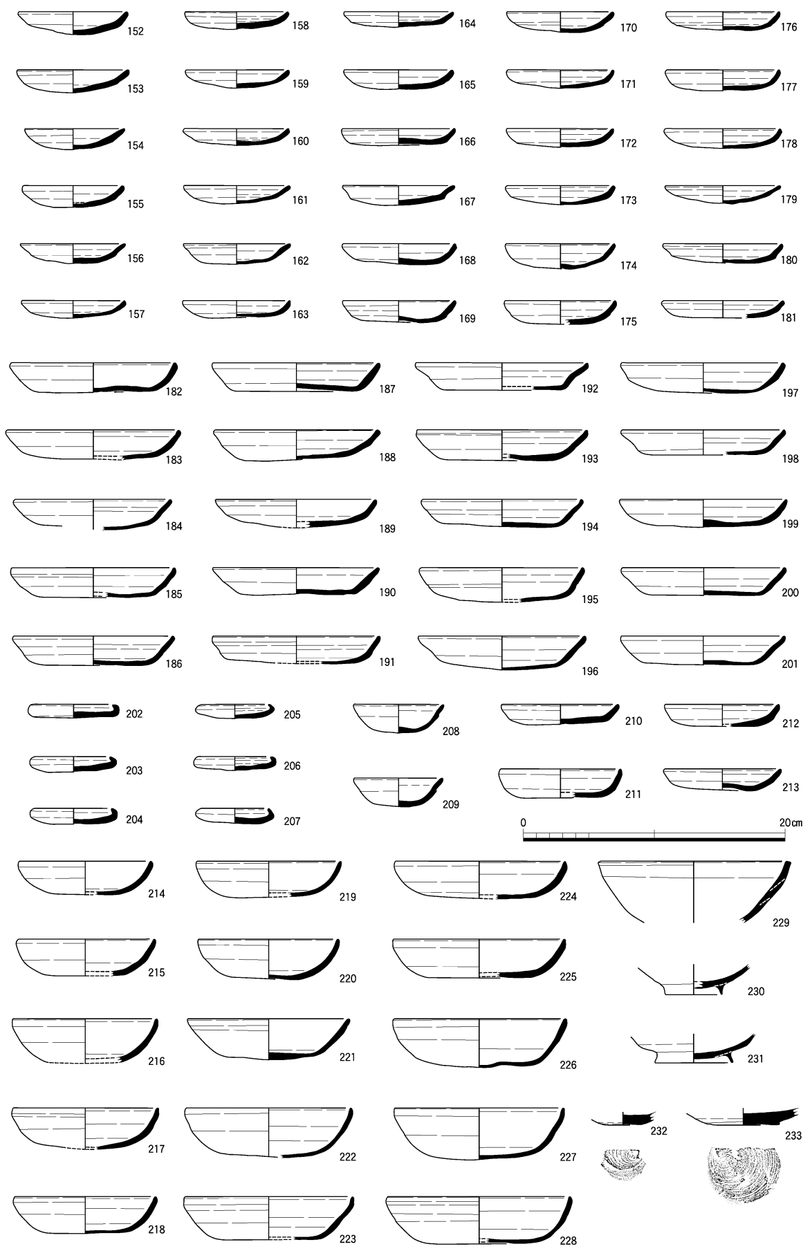
土器実測図4 (1:4)
