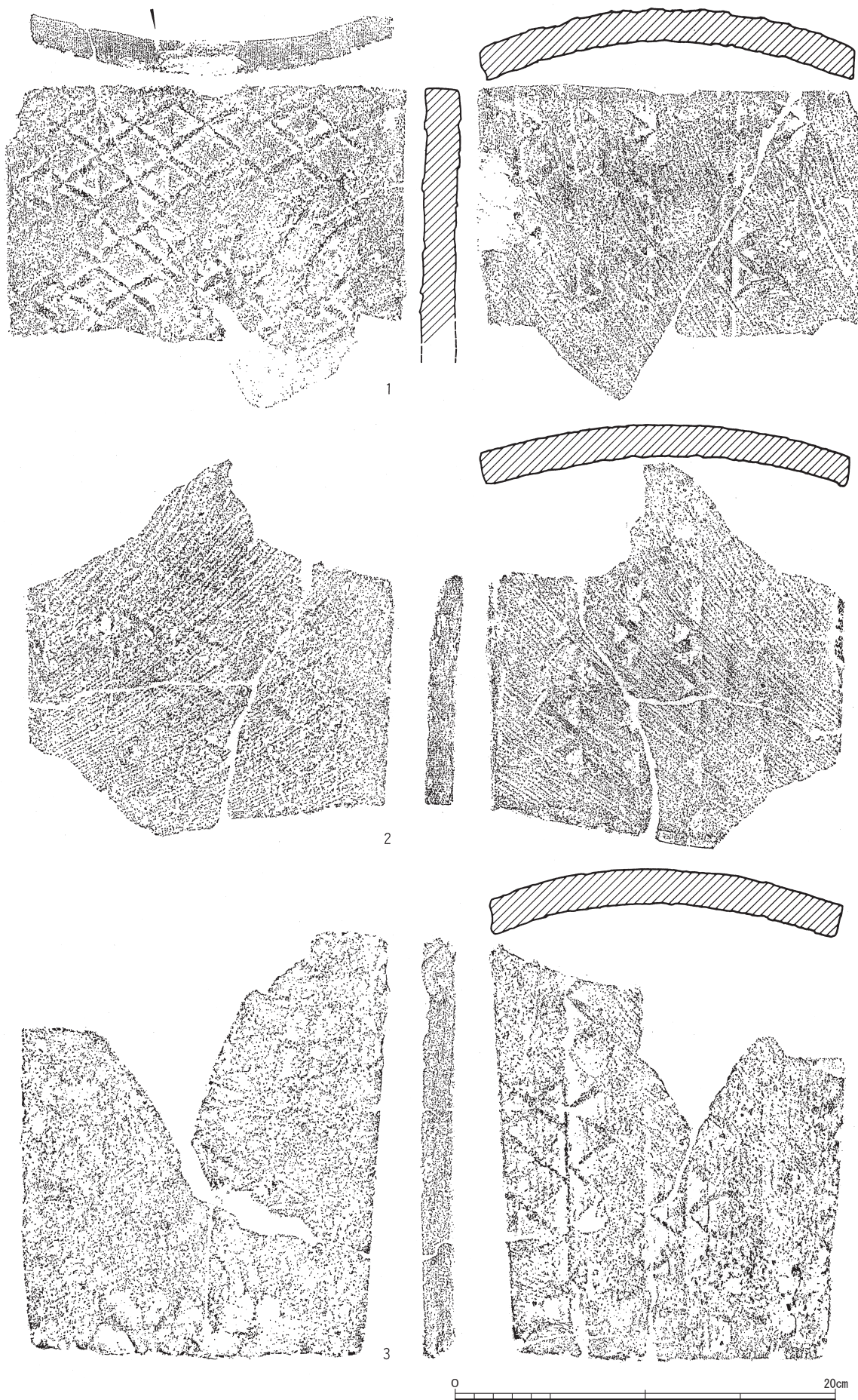
平瓦実測図 1(1:3)
