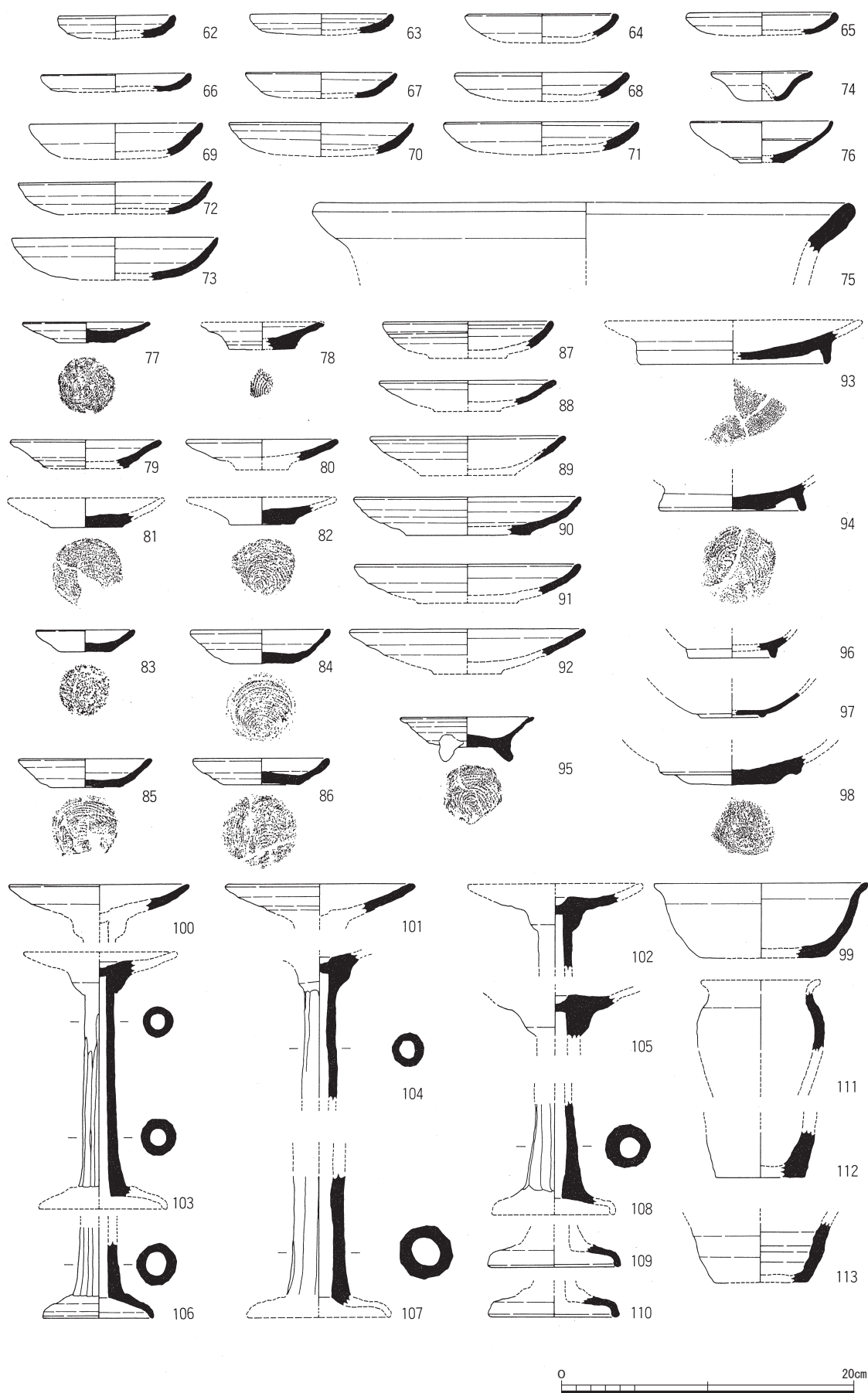
土器実測図2 溝1出土(62~76)・遺物包含層出土(77~113)(1:4)
