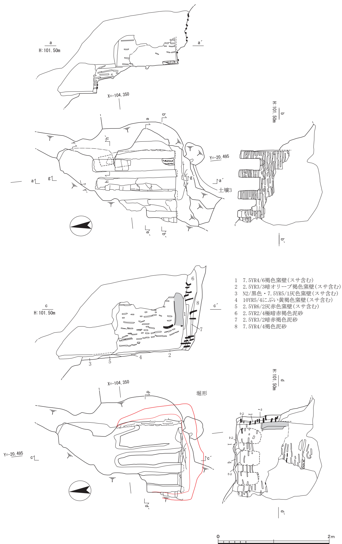
瓦窯実測図(1:40)
