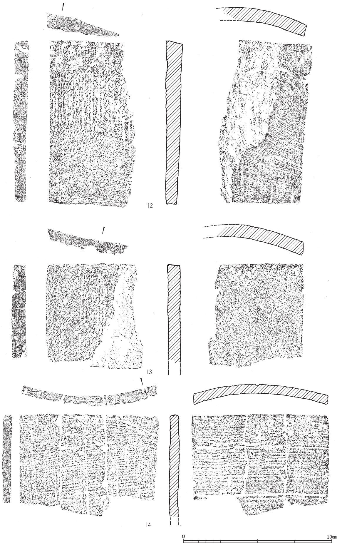
平瓦実測図 5(1:3)
