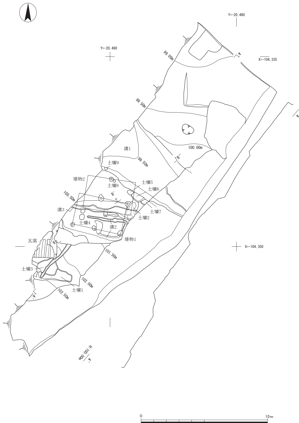
調査区遺構実測図(1:150)
