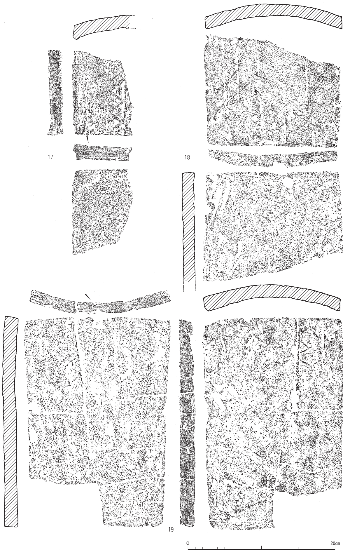
平瓦実測図 7(1:3)
