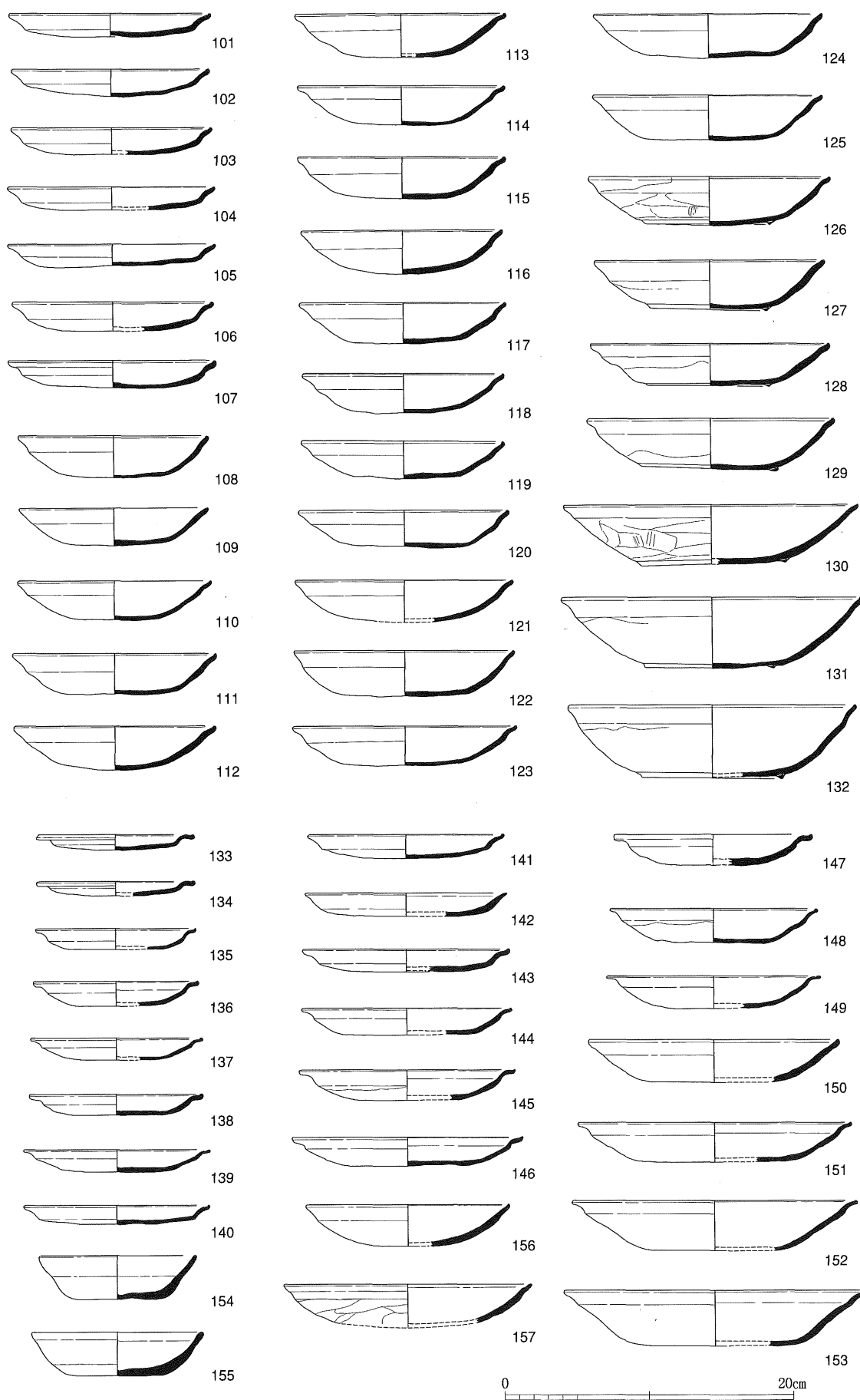
池1出土土師器実測図1 (1/4)
