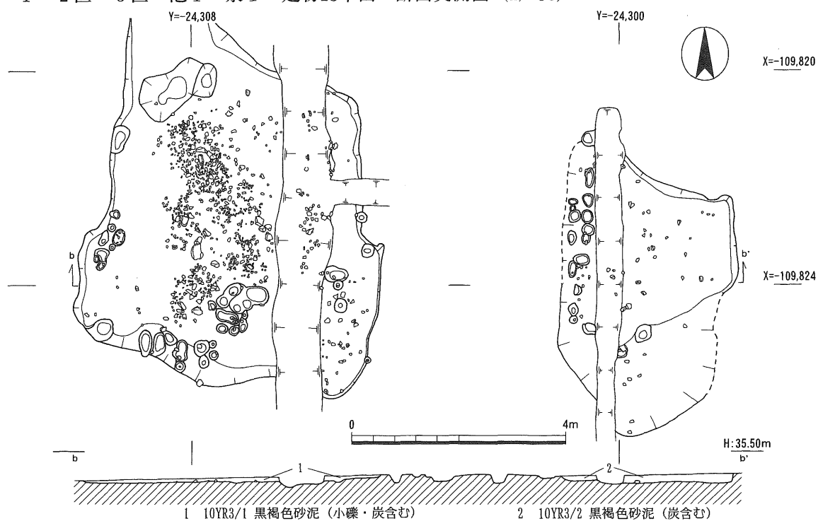
1 2区・3区 池1・泉1・建物13平面・断面実測図 (1/50)
