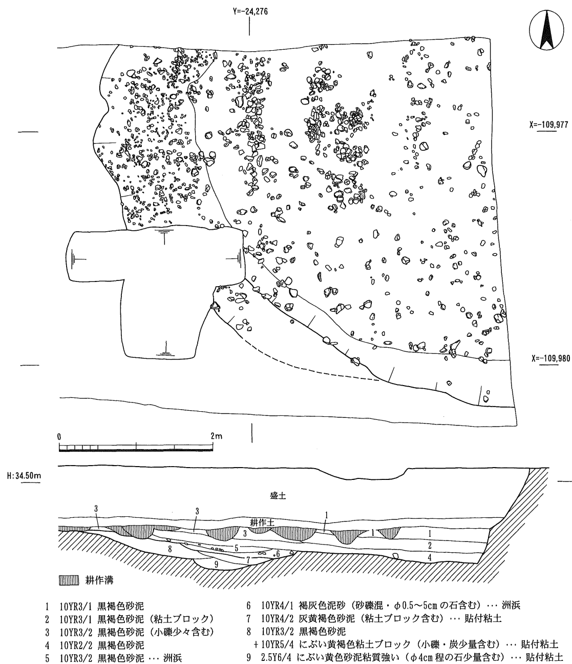
1 第5次調査1区・2区 平面実測図 (1/200)
