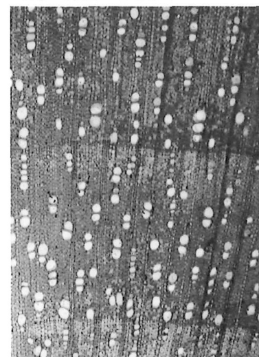
横断面 ————— : 0.5mm 15. 11-15 ムラサキシキブ属
