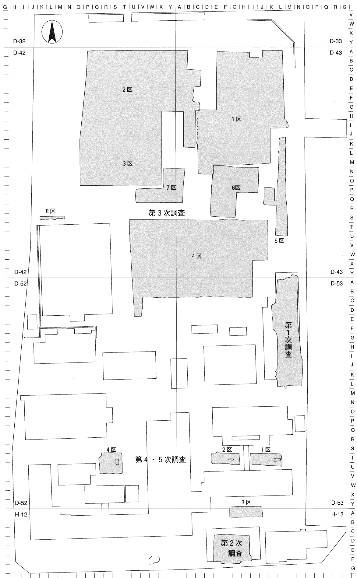
調査対象地の地区割図 (1/1,000)
