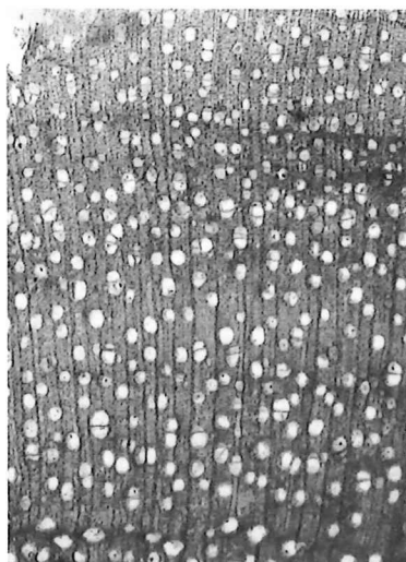
横断面 : 0.5mm 7. 10-22① ヤナギ属
