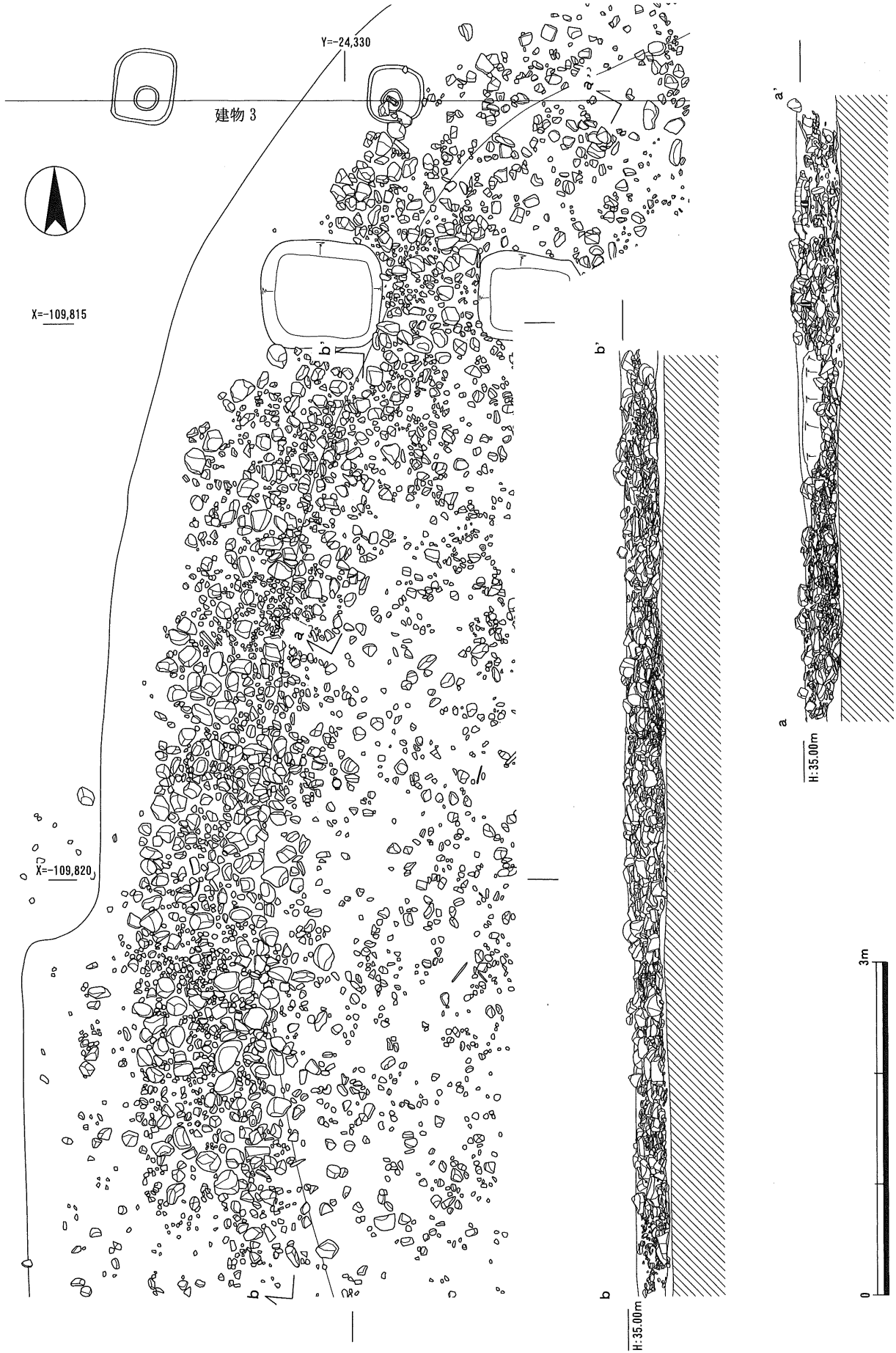
2区・3区 池1西岸部洲浜平面・断面実測図 (1/50)
