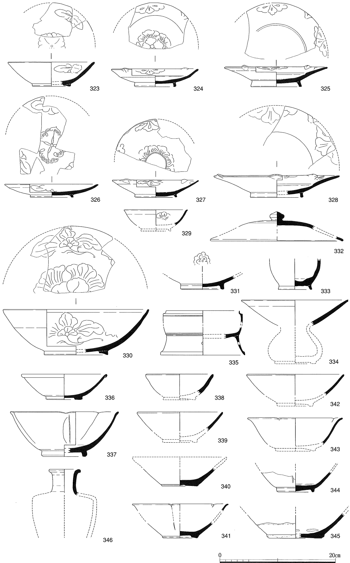
池1出土緑釉陶器・輸入陶磁器(白磁・青磁・褐釉陶器)実測図(1/4)
