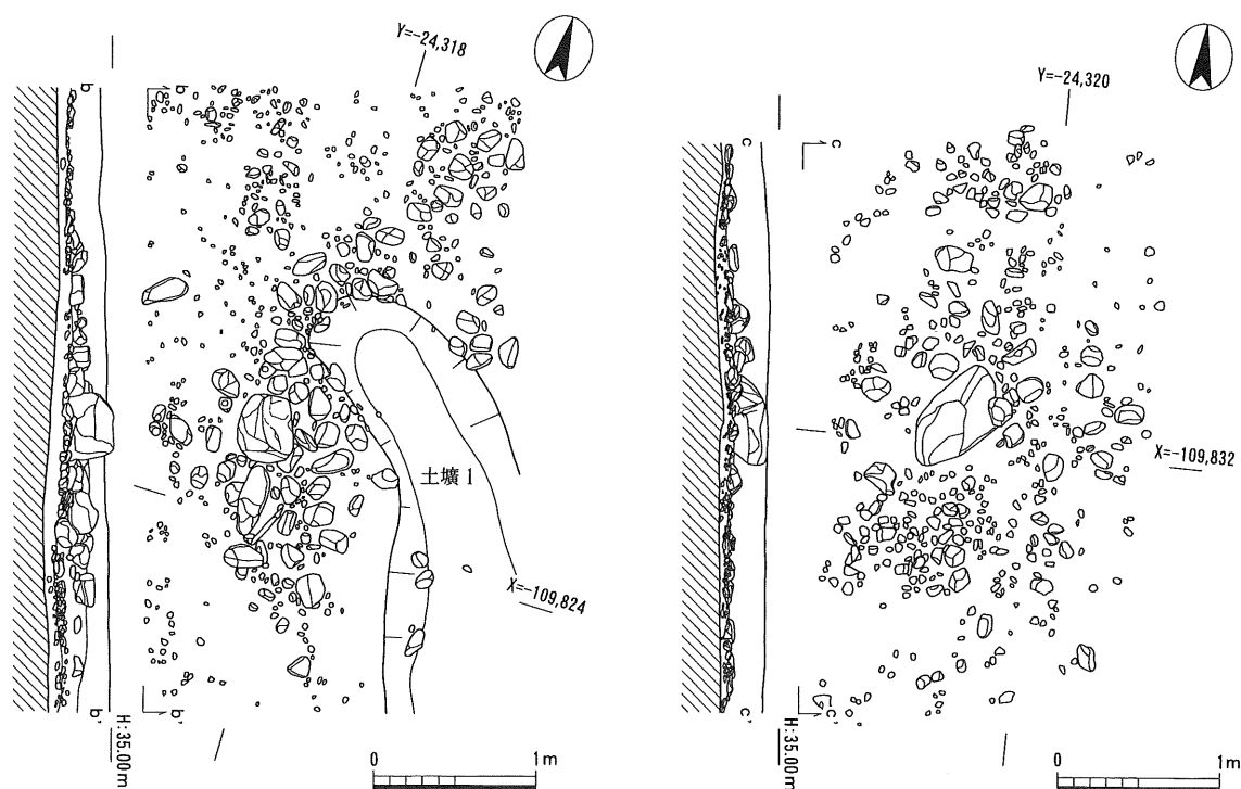
2 同 池1東岸部景石平面・断面実測図 (1/50)
