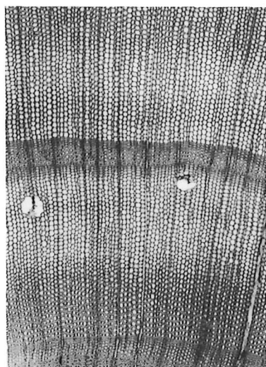
横断面 ————— : 0.5mm 4. 8-15 マツ属複維管束亜属
