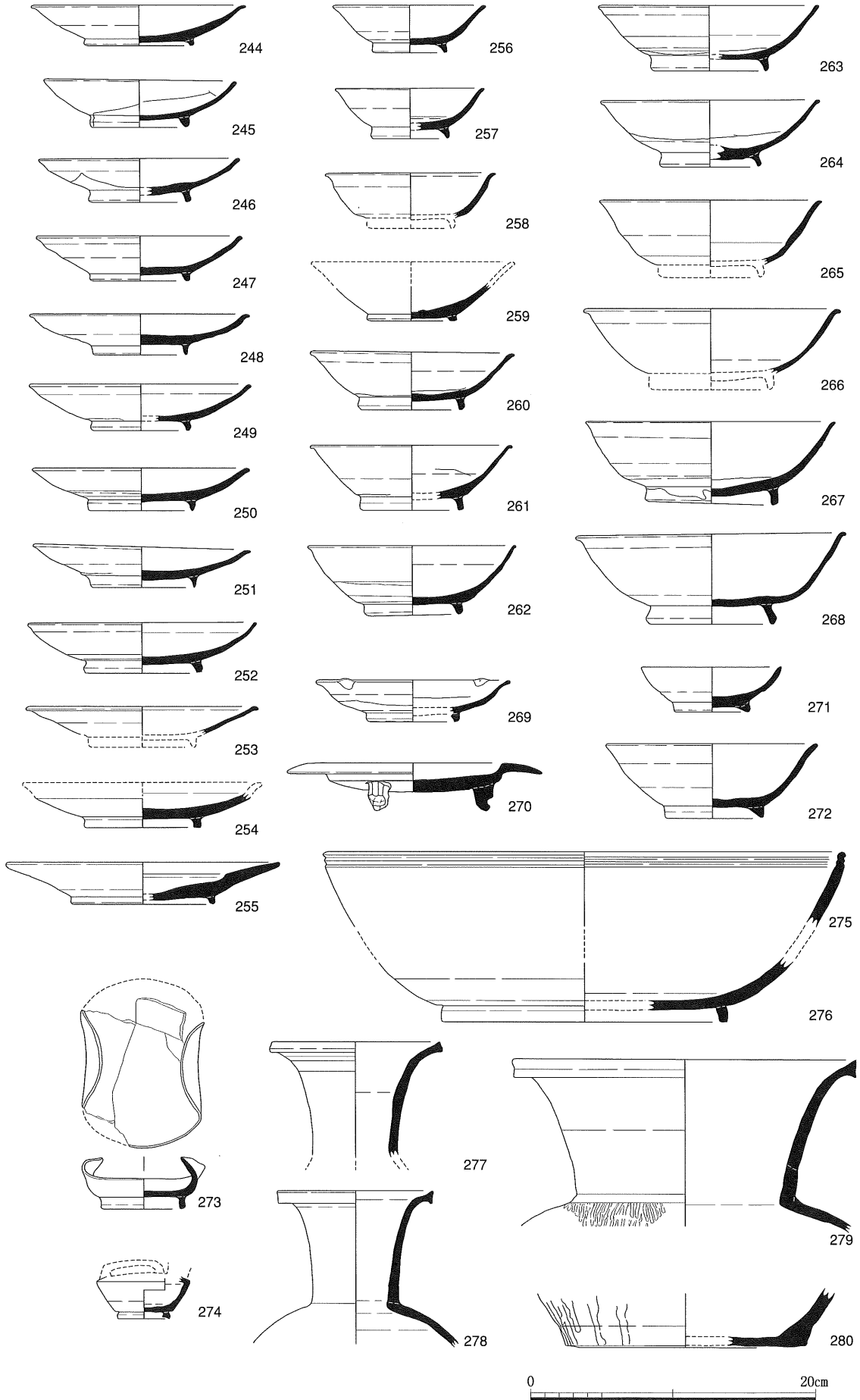
池1出土灰釉陶器実測図(1/4)
