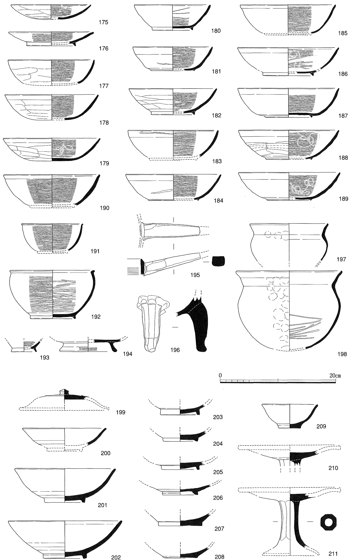
池1出土黒色土器・白色土器実測図(1/4)
