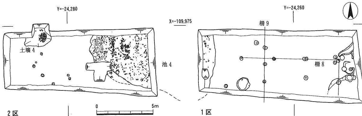
1 第5次調査1区・2区 平面実測図 (1/200)
