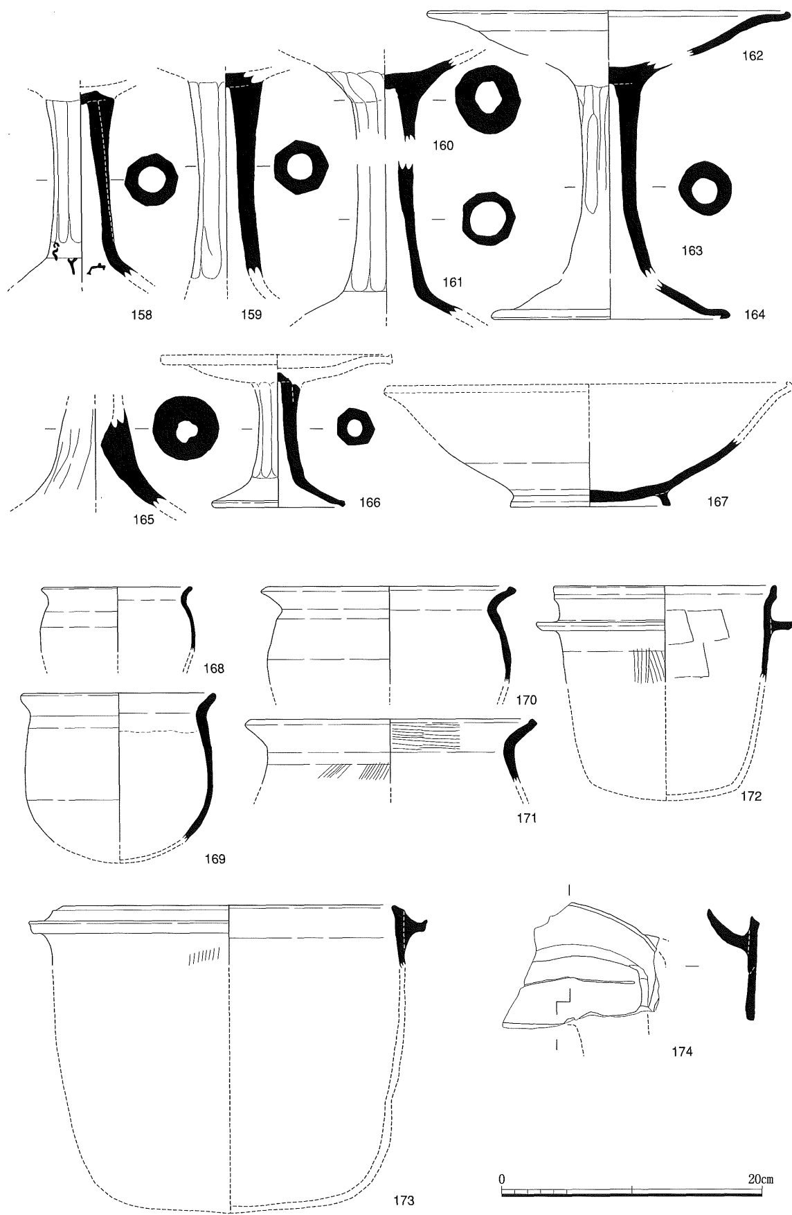
池1出土土師器実測図2 (1 / 4)
