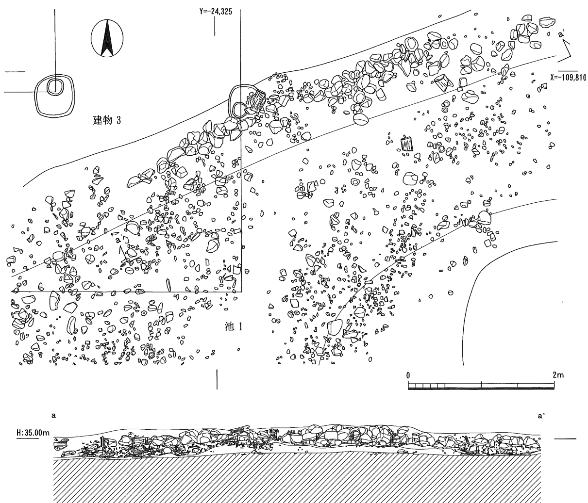
1 2区・3区 池1北岸部平面・断面実測図 (1/50)
