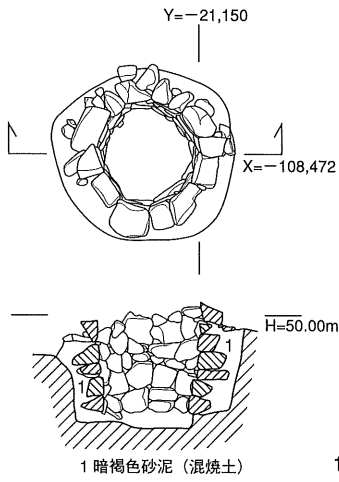
● E区井戸 E 210
