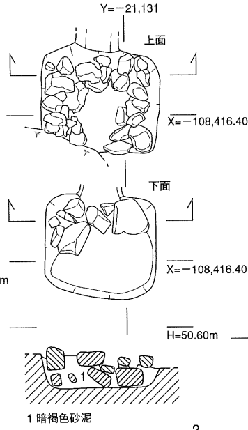
⊙ A区石組土塙A97
