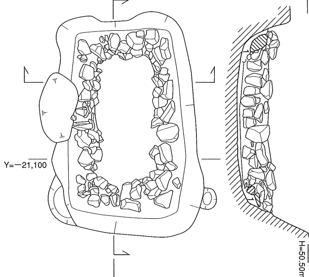
1 D区井戸D296実測図
