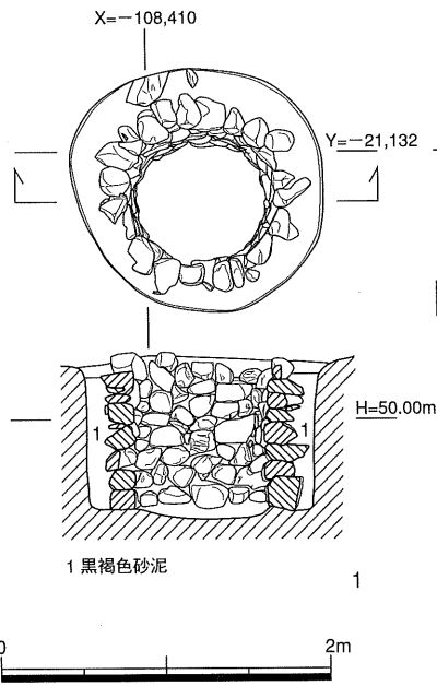
⊙ A区石組土塙A6
