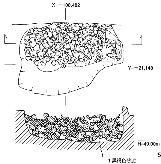
⊙ E区石組土壙 E 123
