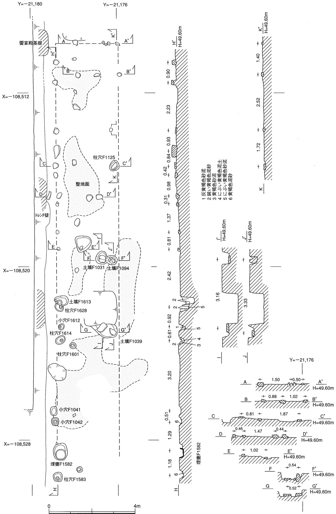
F区建物F2666実測図
