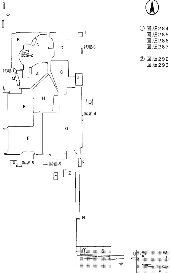
3 S区西部・V・W区平面図配置図
