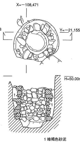
⊙ E区石組土壙 E 123
