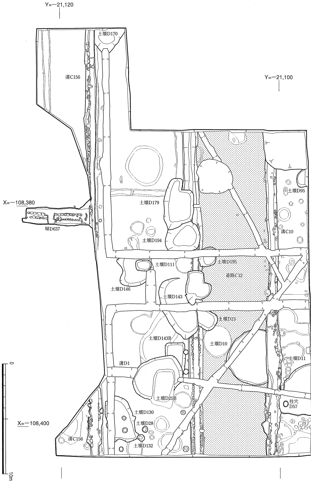
D区江戸時代後期遺構平面図
