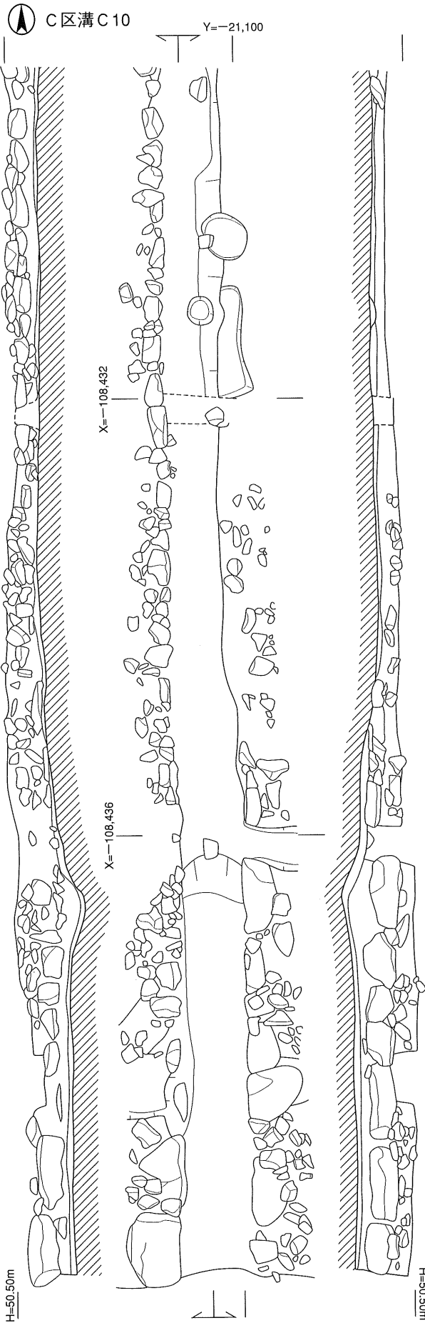
1 C区溝C10実測図
