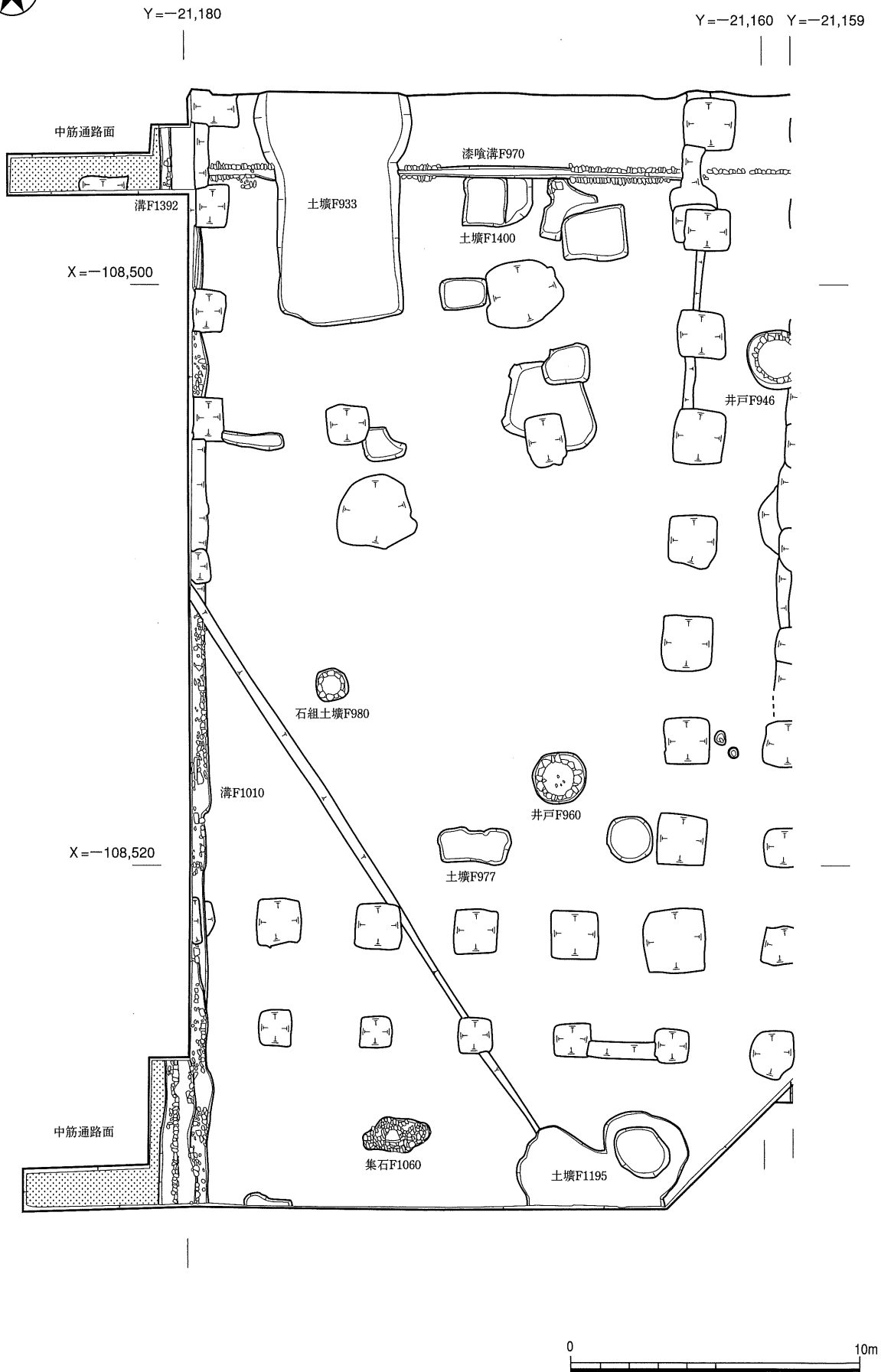
F区西部江戸時代後期遺構平面図
