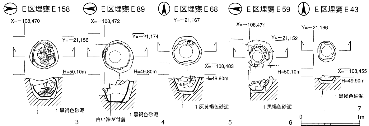
1 E区竈E140実測図 2 E区竈E185実測図 3 E区埋甕E158実測図 4 E区埋甕E89実測図 5 E区埋甕E68実測図 6 E区埋甕E59実測図 7 E区埋甕E43実測図
