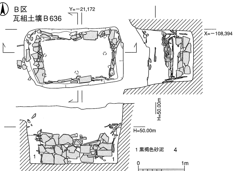
1 B区土壤 B725実測図 2 B区溝 B675実測図 3 B区溝 B678実測図 4 B区瓦組土壤 B636実測図 5 B区埋納土壤 B778実測図
