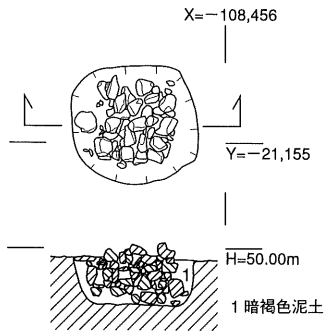
⊙ E区集石 E 203
