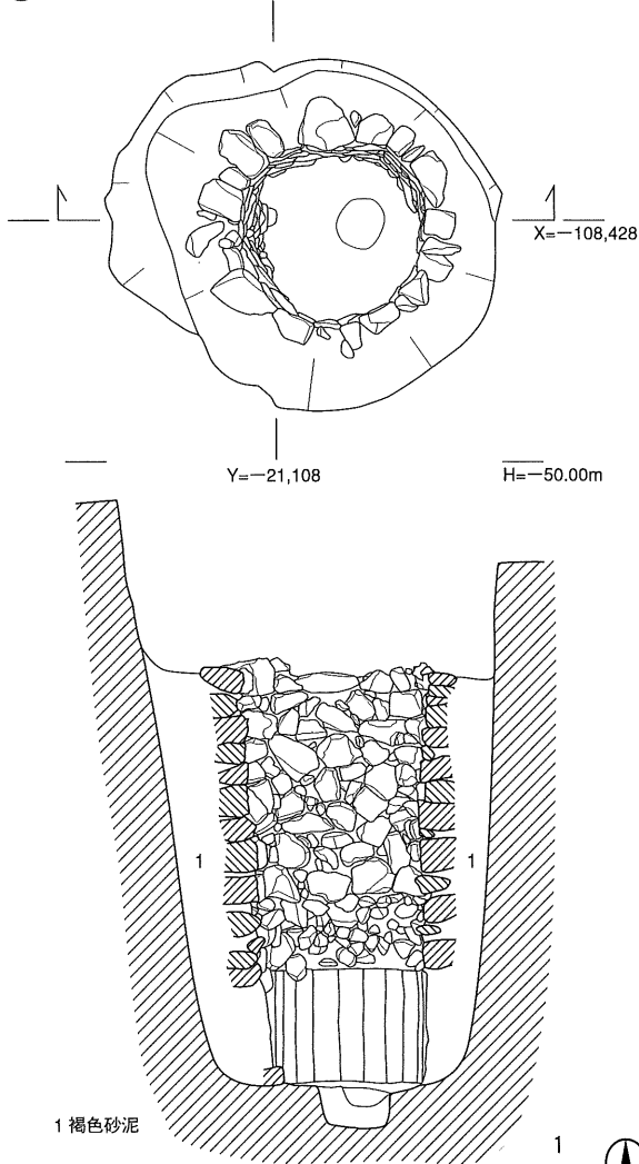
① C区井戸C660
