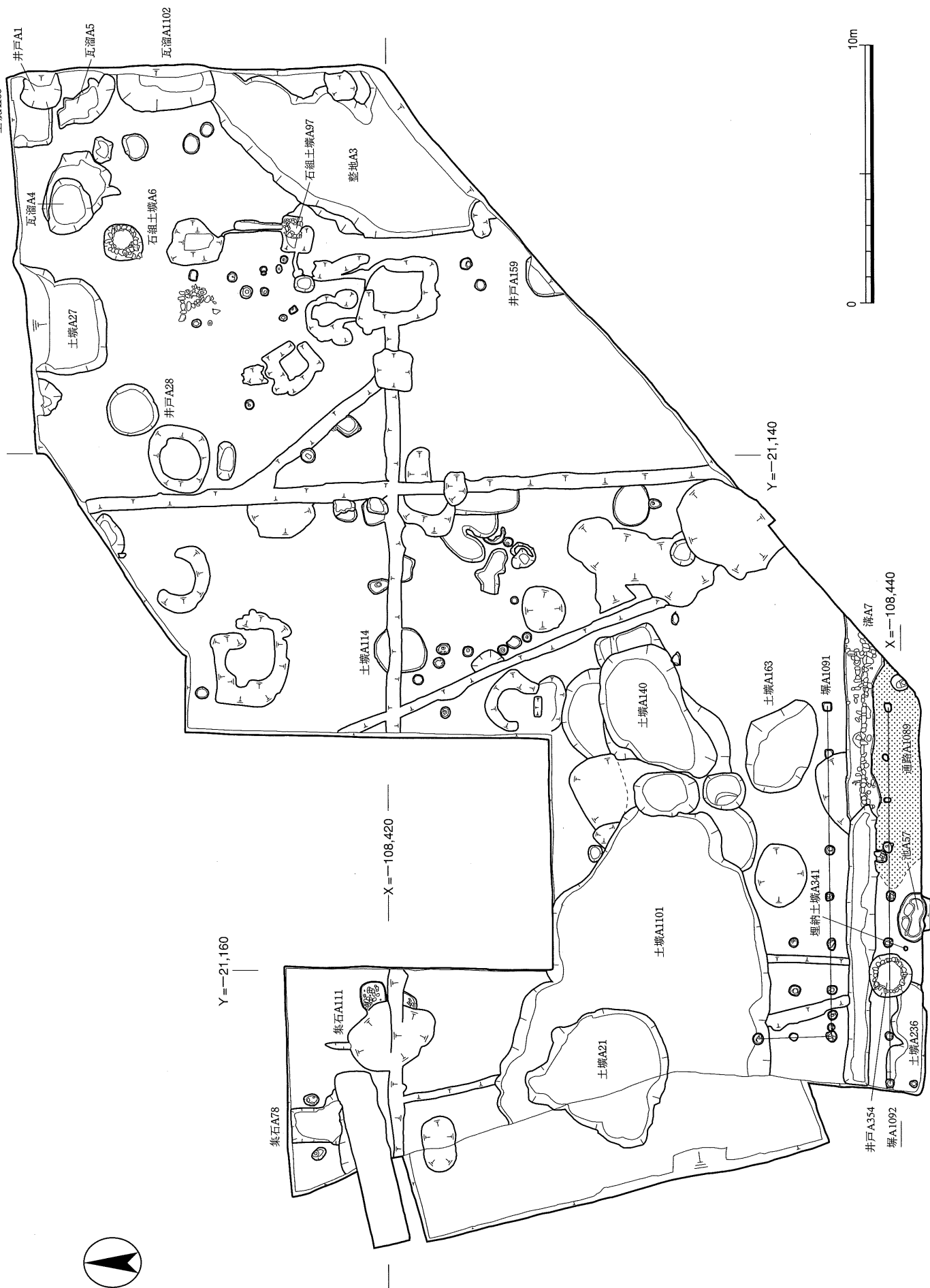
A・M区江戸時代後期遺構平面図
