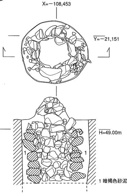
● E区井戸 E 210
