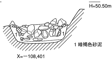
● D区穴蔵D200
