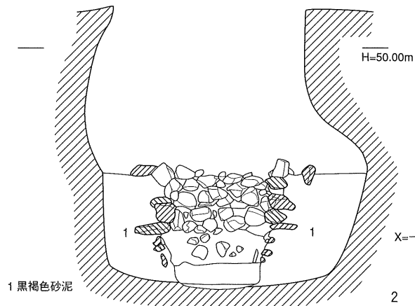
1 D区井戸 D535実測図 2 D区井戸 D438実測図 3 D区井戸 D318C実測図 4 D区石組土塙 D346実測図 5 D区塀 D303実測図
