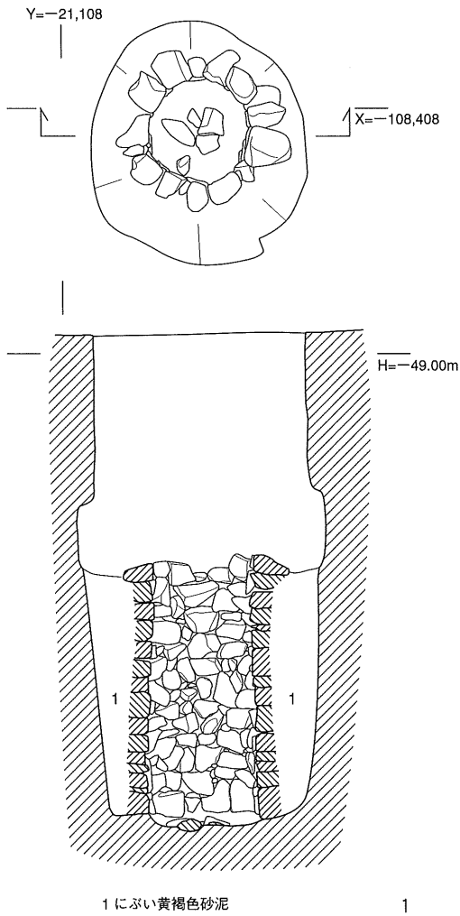
① C区井戸C661
