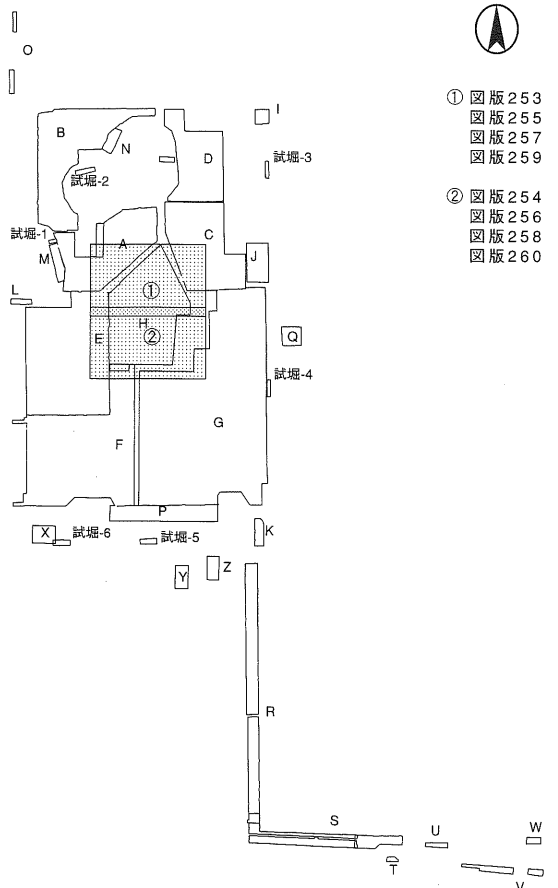
4 H区平面图配置图
