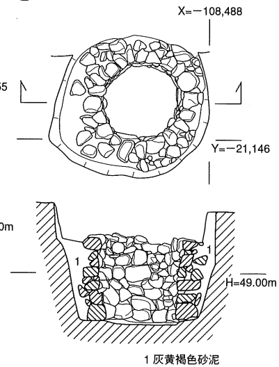
⊙ E区石組土壙 E 371
