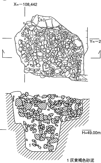
⊙ E区集石 E 134
