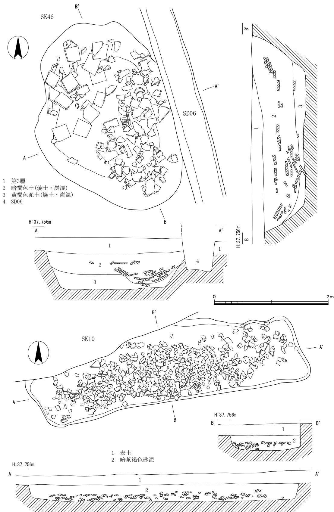
土壌実測図 (SK10・46) (1:40)
