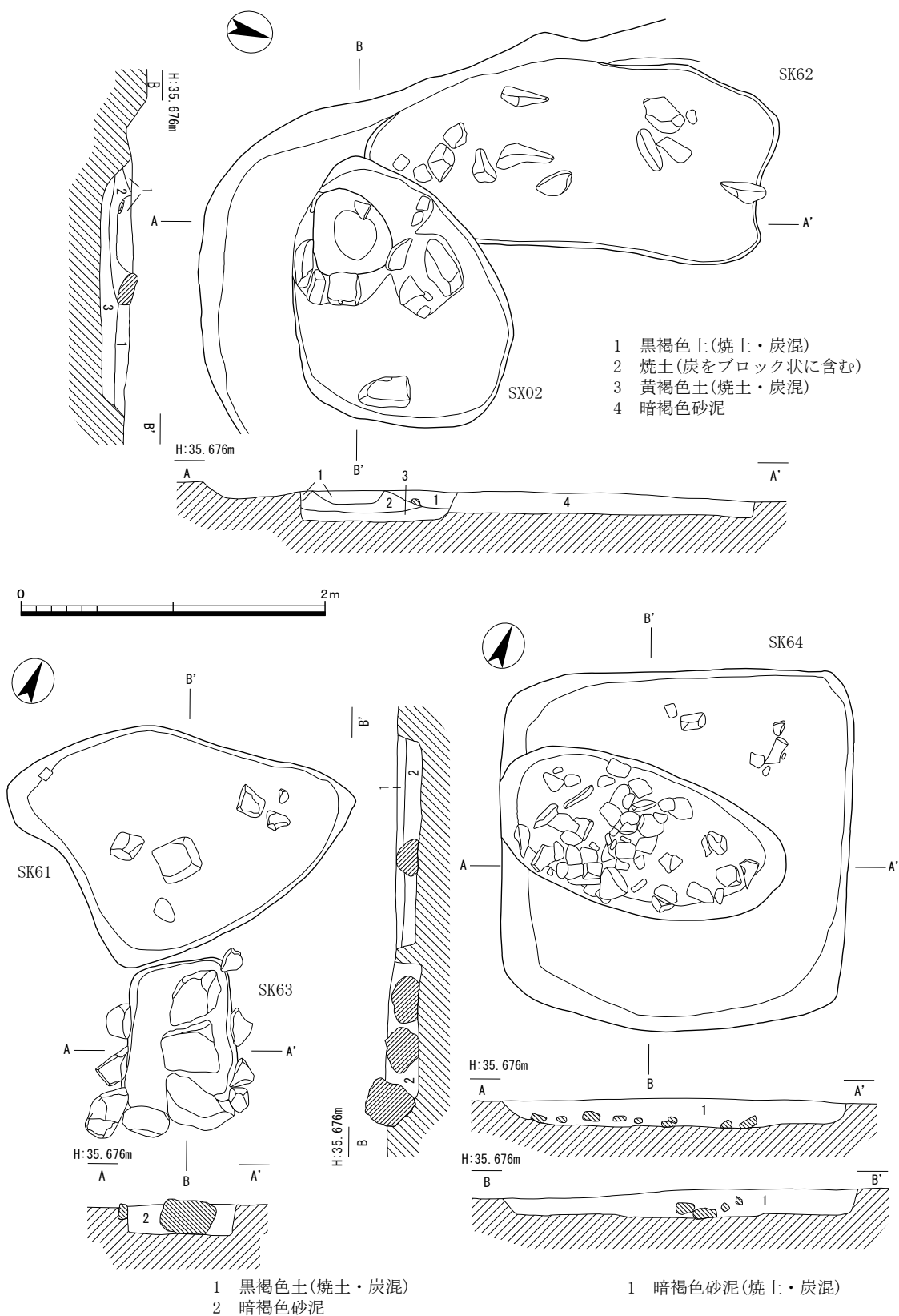
土壌実測図 (SK61・62・63・64、SX02) (1:40)
