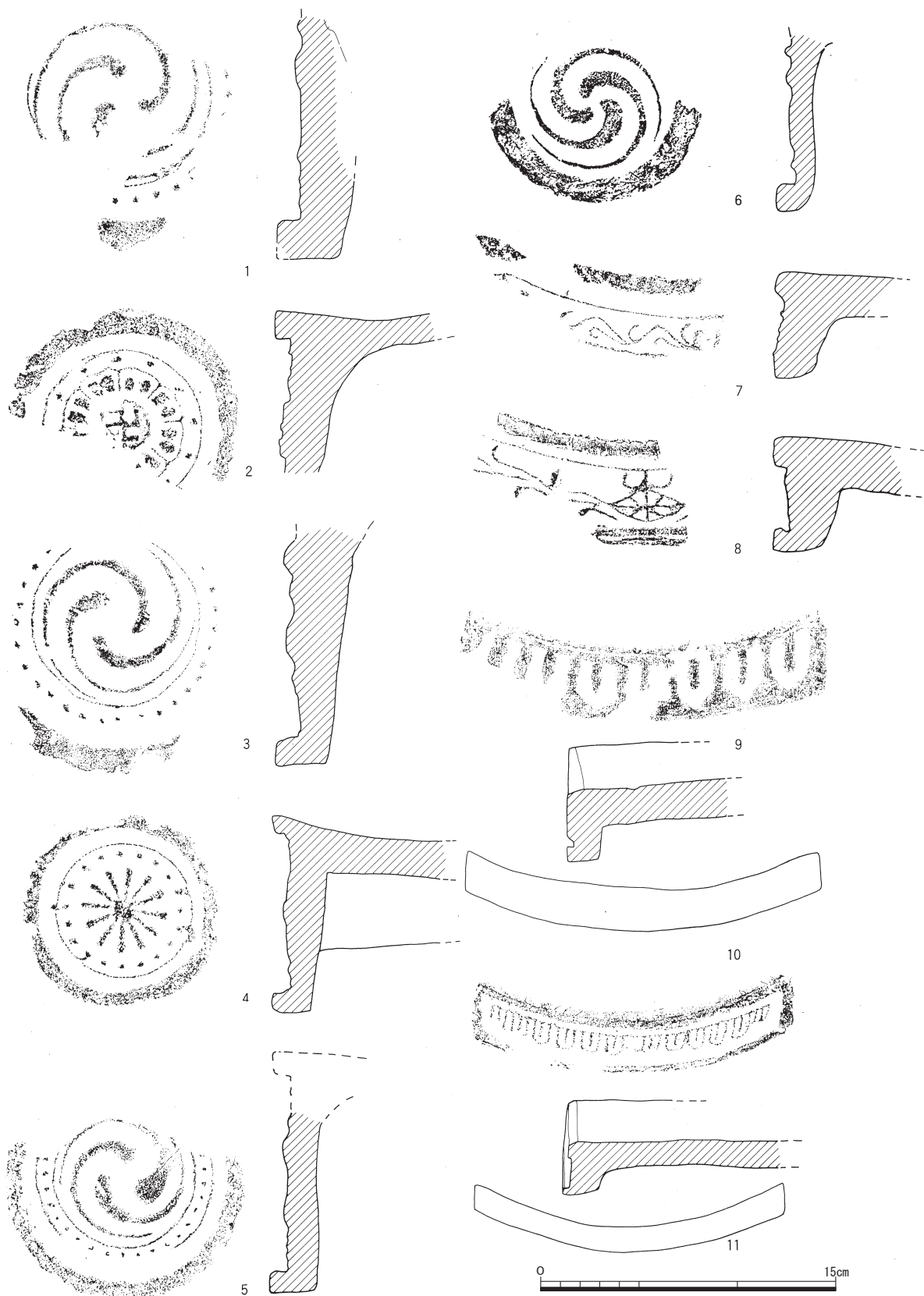
SD12 軒丸瓦 1・2・6・軒平瓦 7・8 SE1 軒丸瓦 5 SK14 軒丸瓦 3 軒平瓦 9 SX2 軒丸瓦 4 軒平瓦 10 (1:3)
