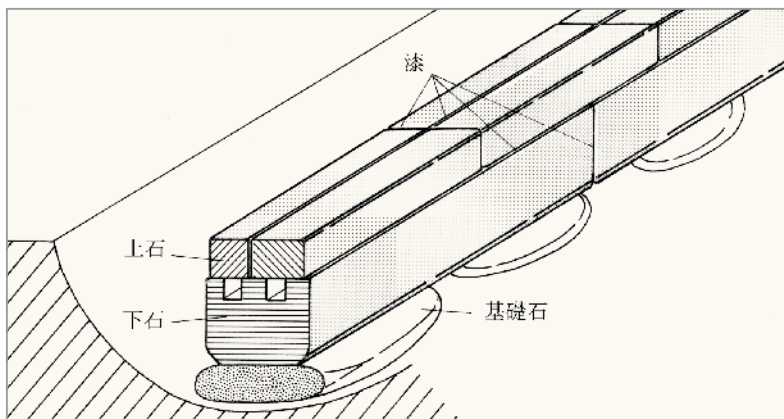
石製導水施設の模式図
