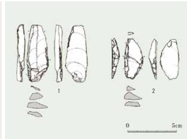
図2 写真3-1・3-2ナイフ形石器の実測図
