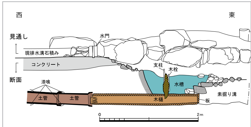
図2 排水施設実測図
