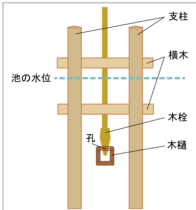
図1 排水施設模式図
