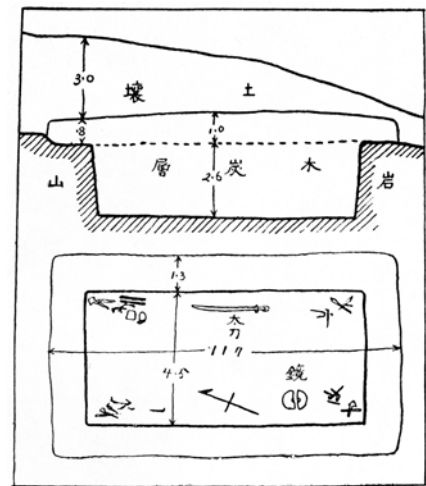
図2 西野山古墓墳実測図（図1-3） 『京都府史蹟勝地調査会報告 第2冊』 大正9年 京都府
