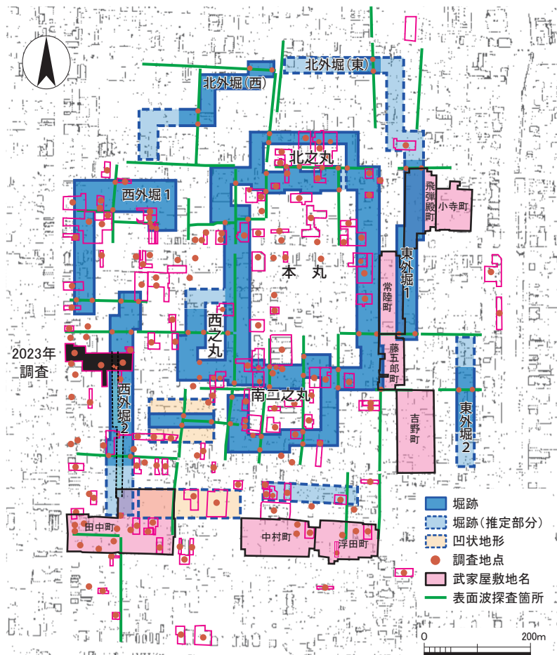
図1 これまでの聚楽第復元図(ただし、外堀の有無は不明)
