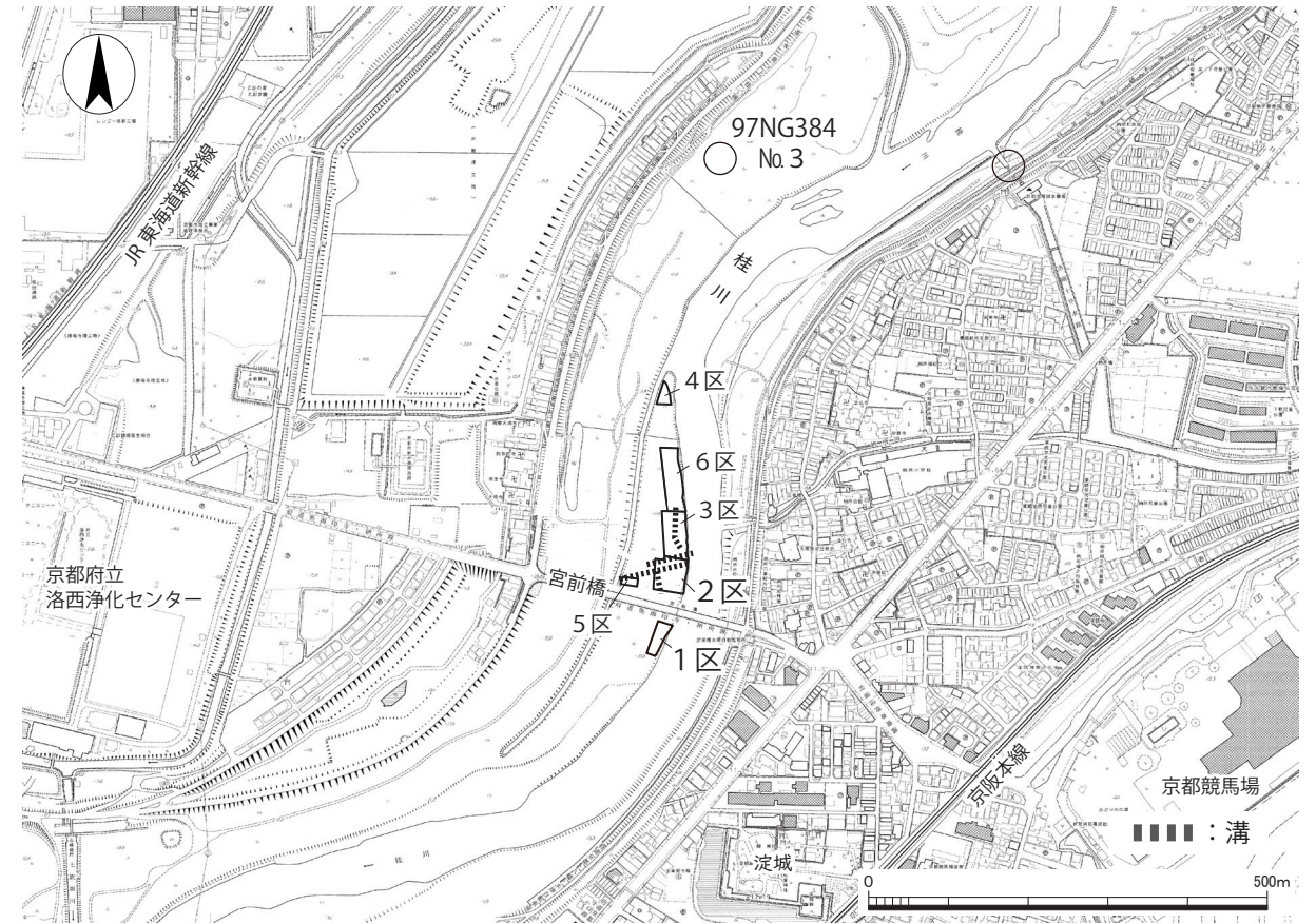
図 23 淀水垂大下津町遺跡調査位置図 (1 : 10,000)
