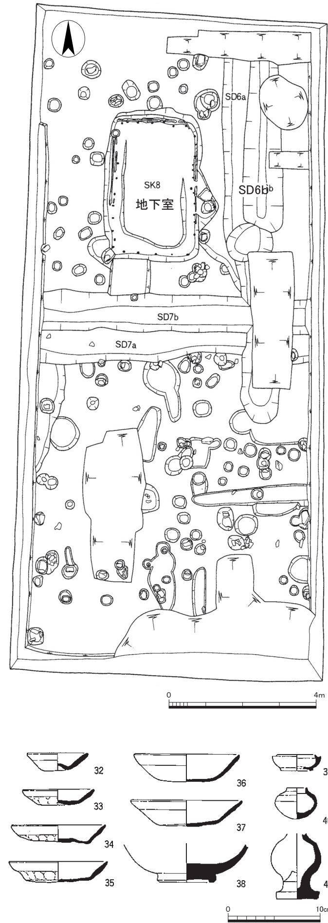
図7 第130次調査平面図 (1 : 100) SD6b出土土器 (1 : 4)
