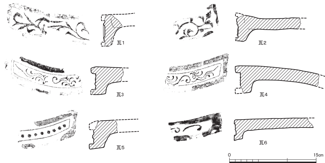
図 17 富ノ森城跡出土軒平瓦実測図 (1 : 4)
