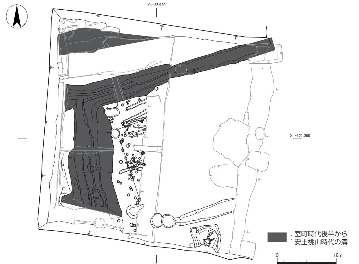
図 24 2区 遺構平面図 (1 : 400)
