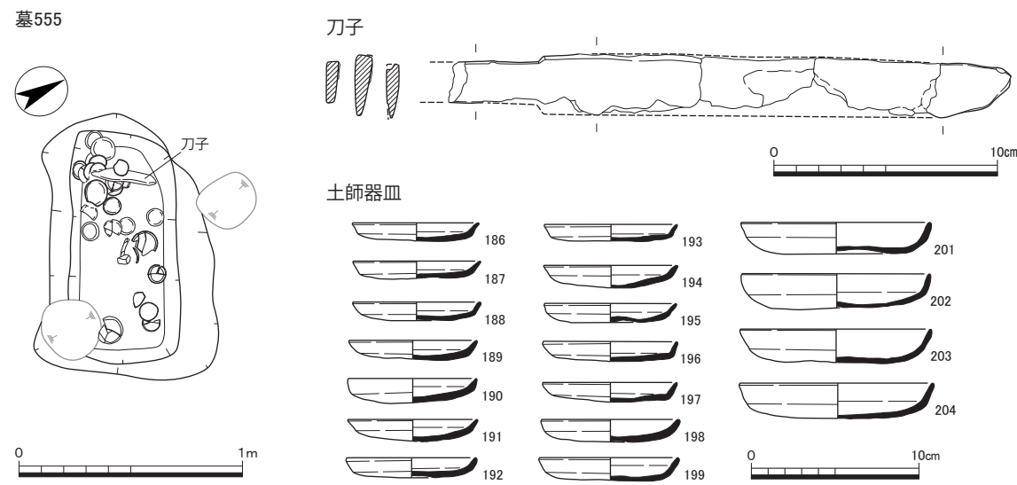
図 15 墓 555 遺構実測図 (1 : 30)・遺物実測図 (1 : 3、1 : 4)
