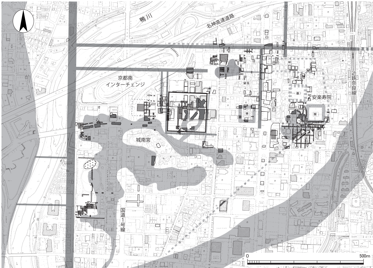
図2 平安時代後期から鎌倉時代遺構図 (1 : 10,000)
